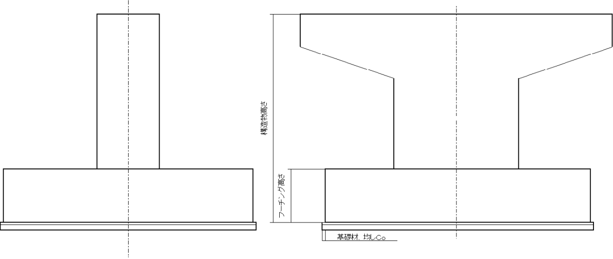
T型橋脚
