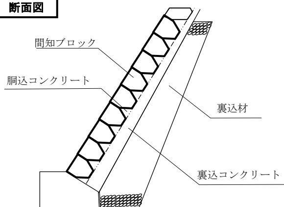
断面図
