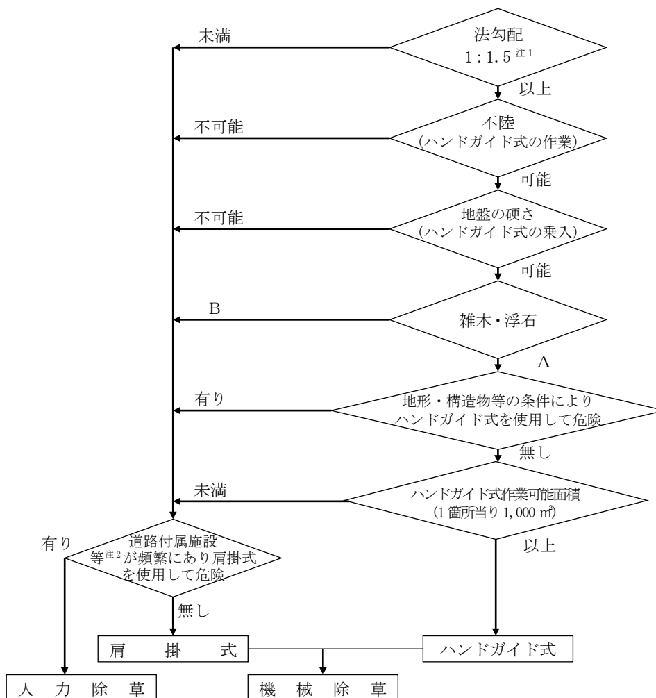
工法の選定フロー
