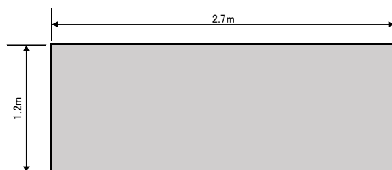
帯鋼補強土壁（２）正面図
