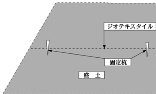
図C 普通敷設工法（壁面材なし）参考図
