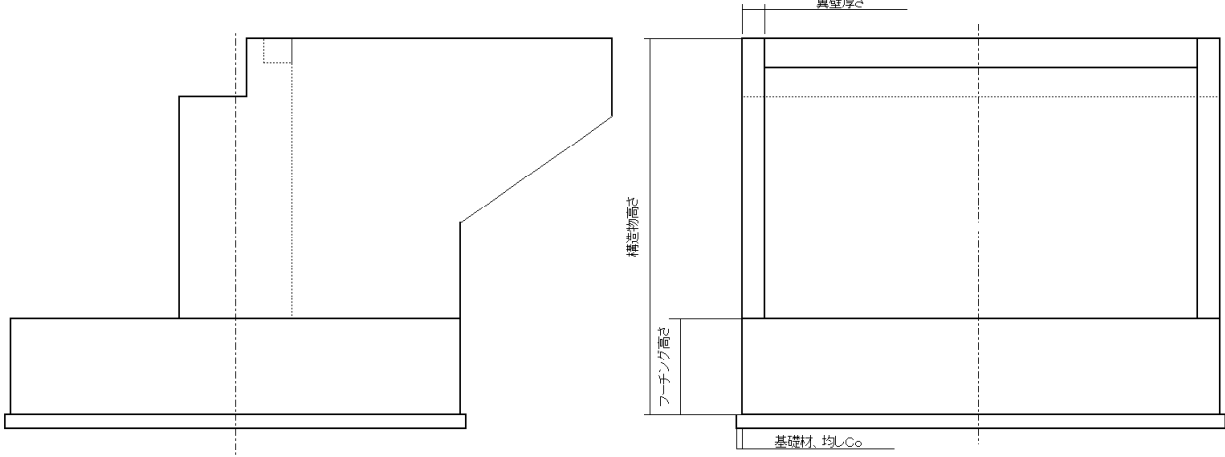
逆T式橋台
