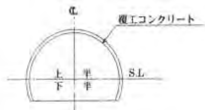
図 1.1 加背割図
