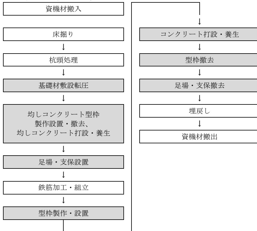
図 2.1 施工フロー
