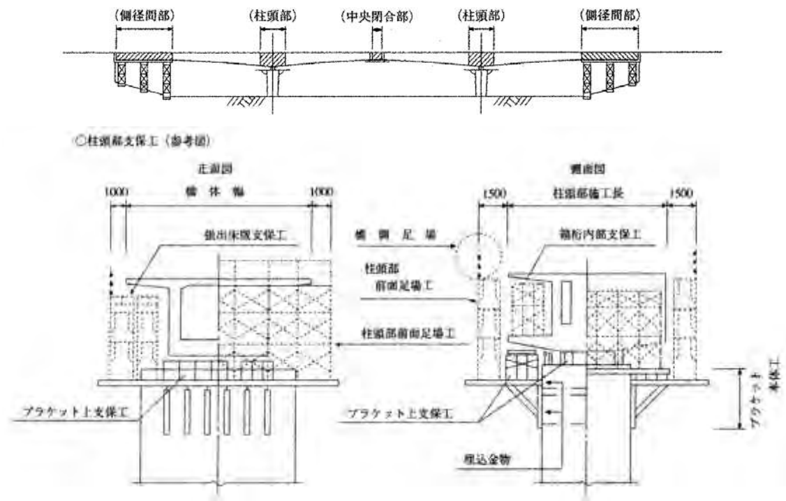
〈ブラケット式支保工〉
