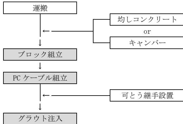
図 2-1 施工フロー
