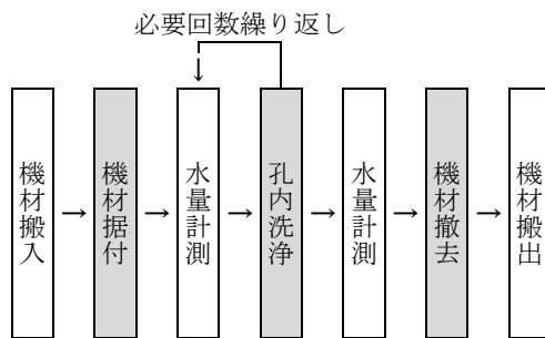
図 2-1 施工フロー
