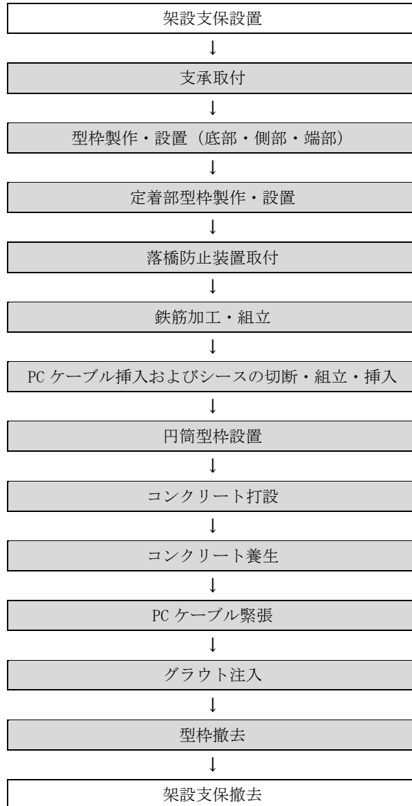
図 2.1 施工フロー
