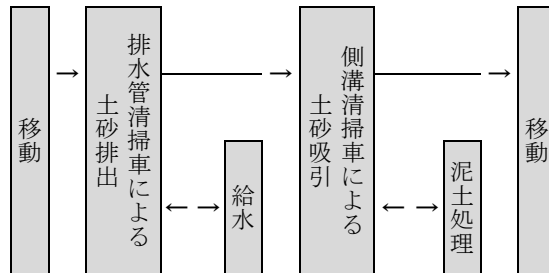
図 2-1 施工フロー
