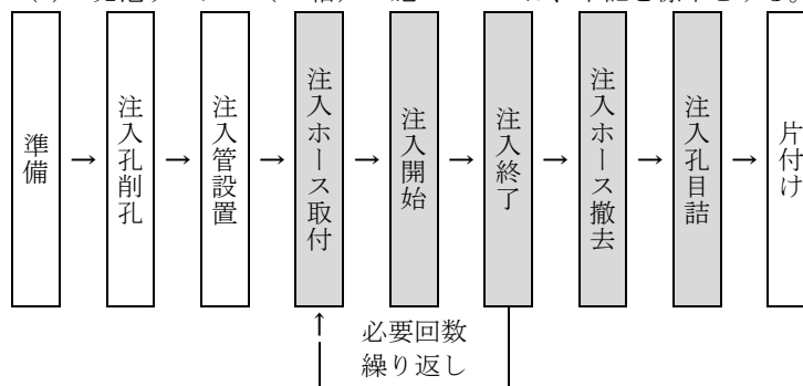
図 2.2 施工フロー
