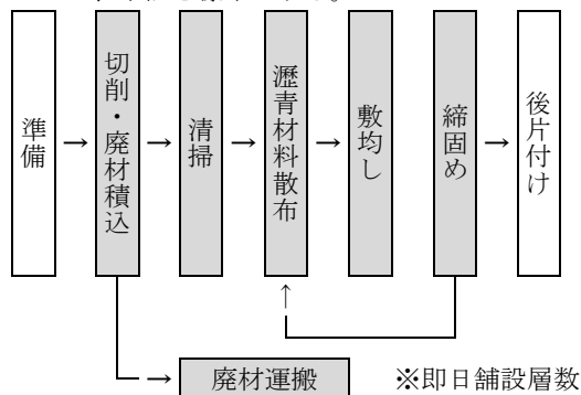
図 2.1 施工フロー
