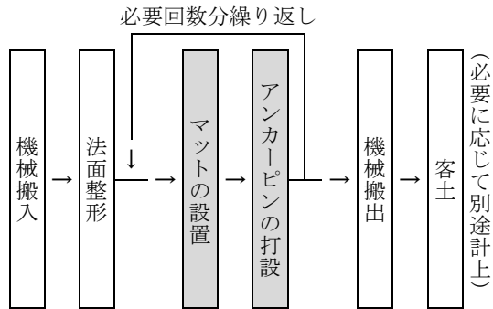
図 2-1 施工フロー
