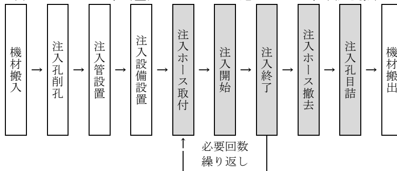
図 2.1 施工フロー
