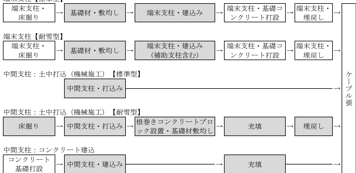
図 2-1 施工フロー
