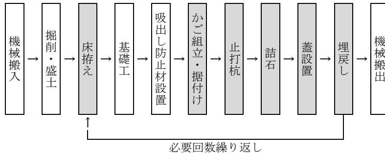
図 2-1 施工フロー
