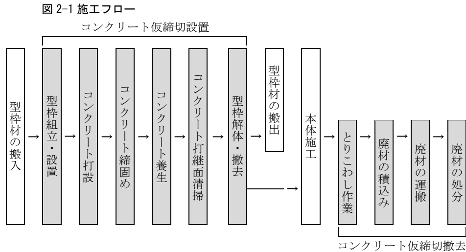
図 2-1 施工フロー
