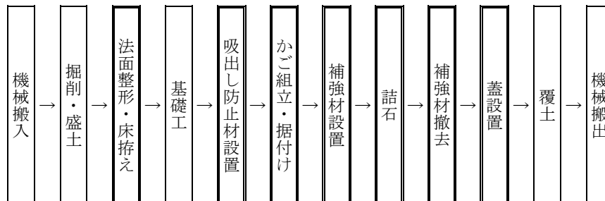
図 2-1 施工フロー
