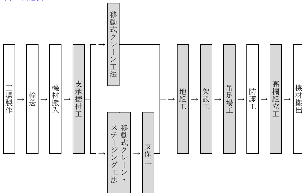
図 2-1 施工フロー
