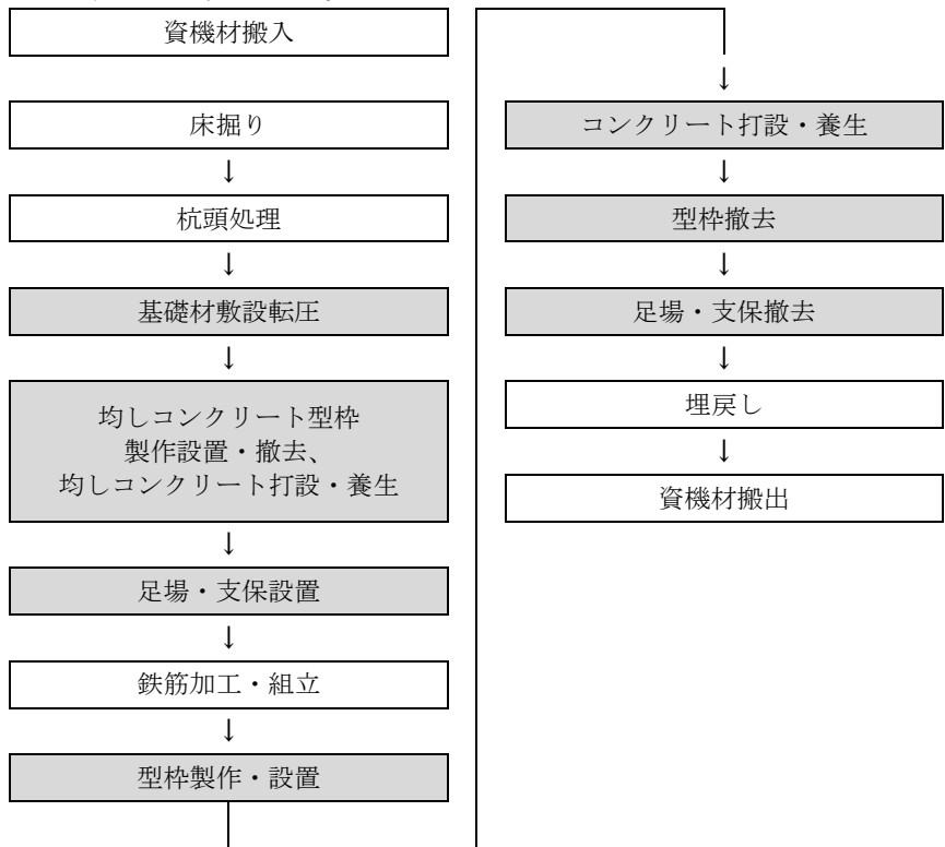
図 2.1 施工フロー
