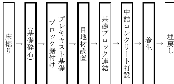
図 2-1 施工フロー
