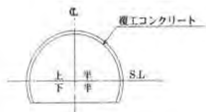
図 1.1 加背割図
