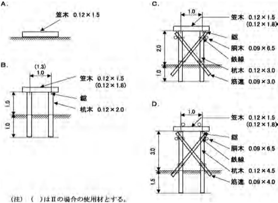
図 5-2 受枠の構造図
