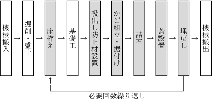
図 2-1 施工フロー
