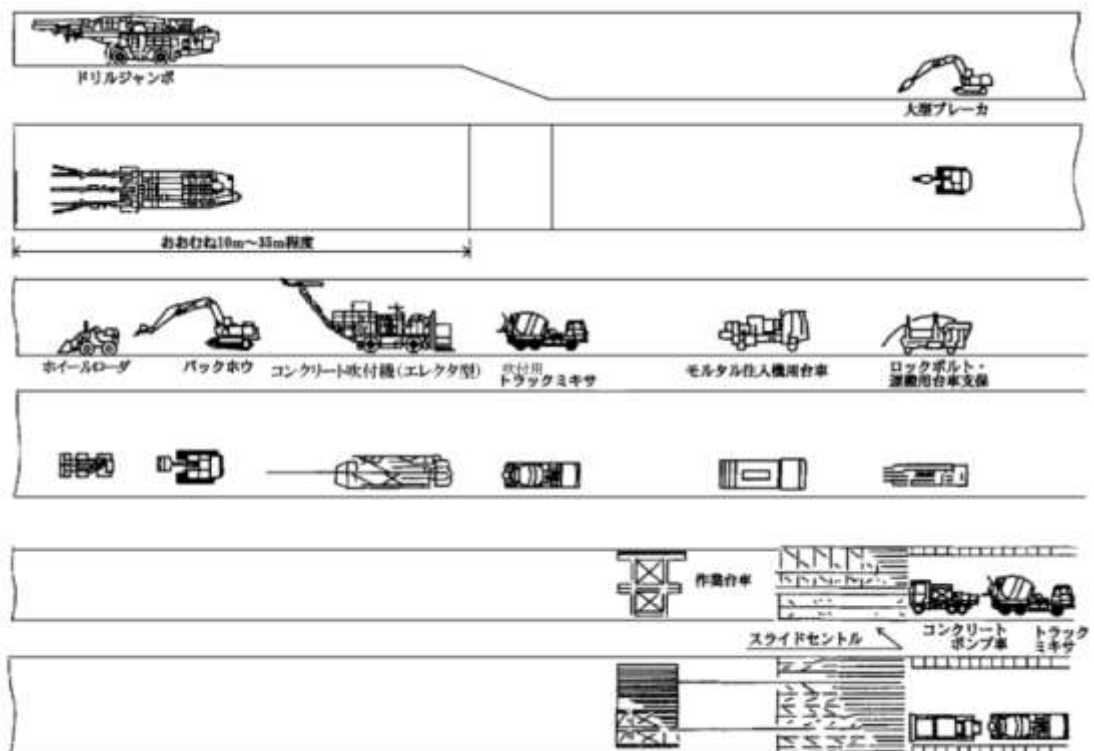
掘削機械配置例 (4) (上半ロックボルト作業時)
