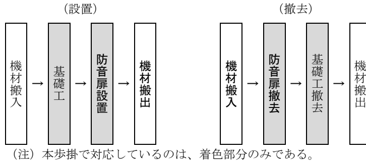
図 2-1 施工フロー
