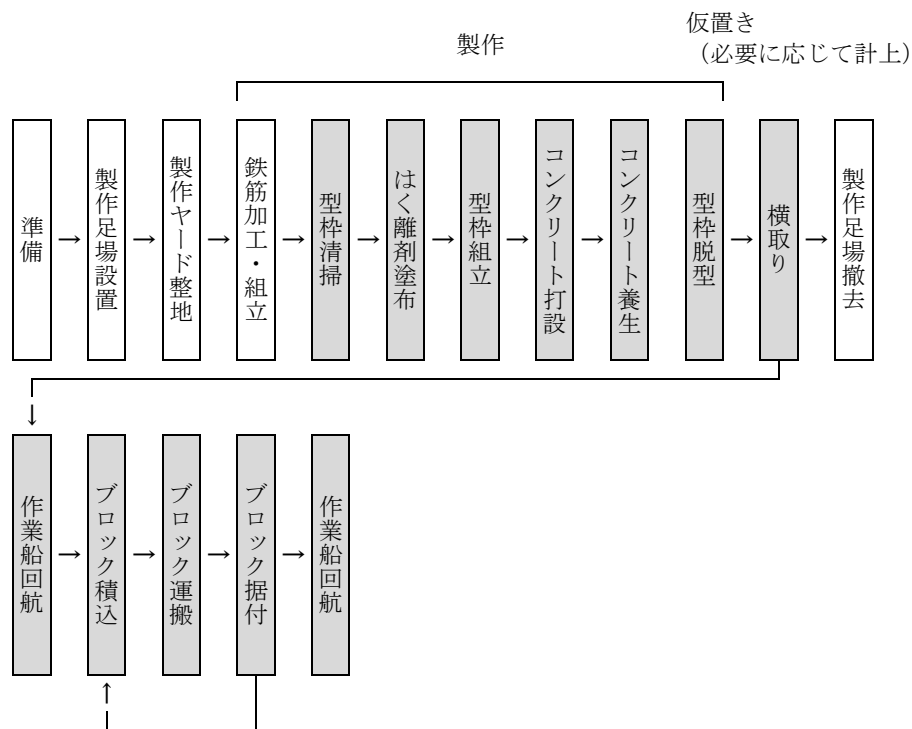
図 2-2 施工フロー
