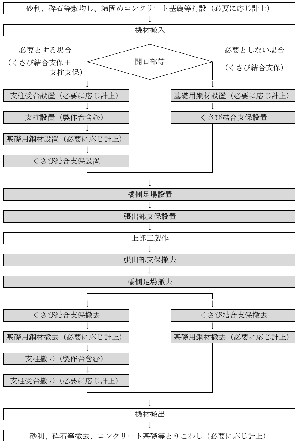
図 2-1 施工フロー
