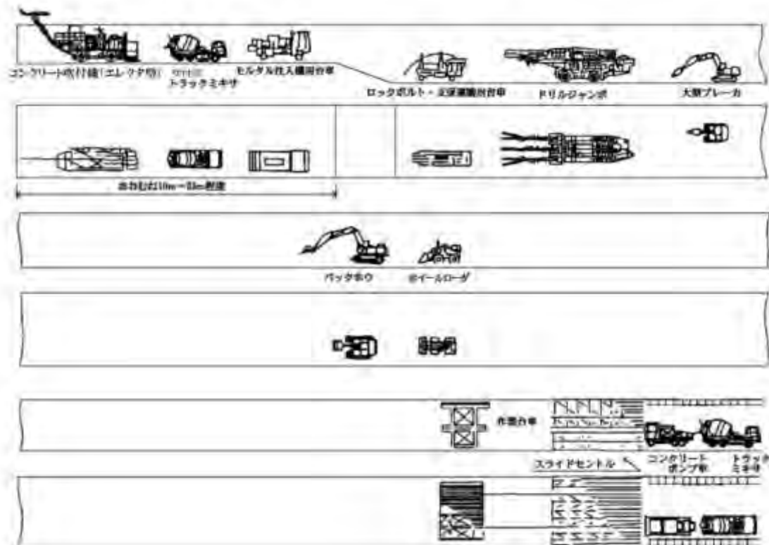
掘削機械配置例 (3) (上半吹付コンクリート作業時)
