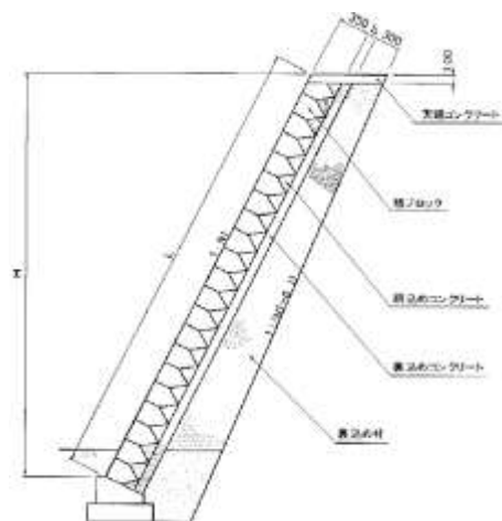
参考図 石積（練石）（複合）の断面図
