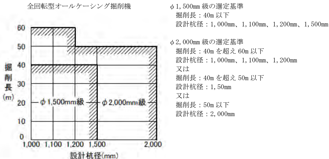
図 3-1 掘削機別選定
