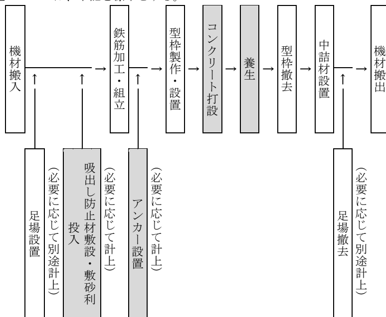
図 2-1 施工フロー
