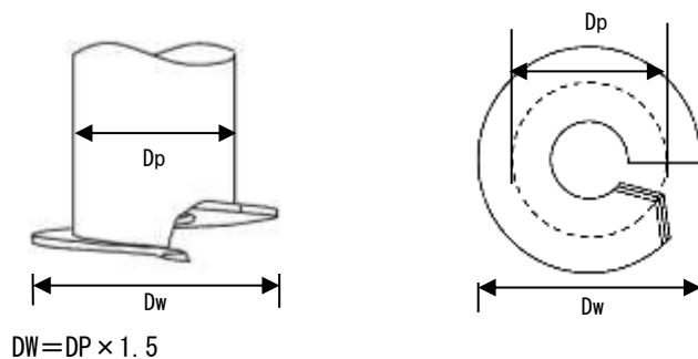
図 1-1 施工図
