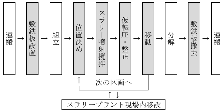
図 2-1 施工フロー
