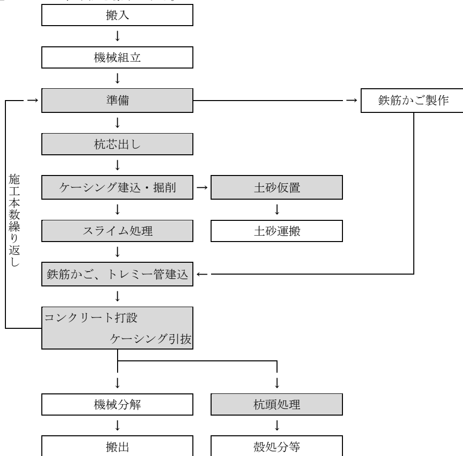
図 2-1 施工フロー
