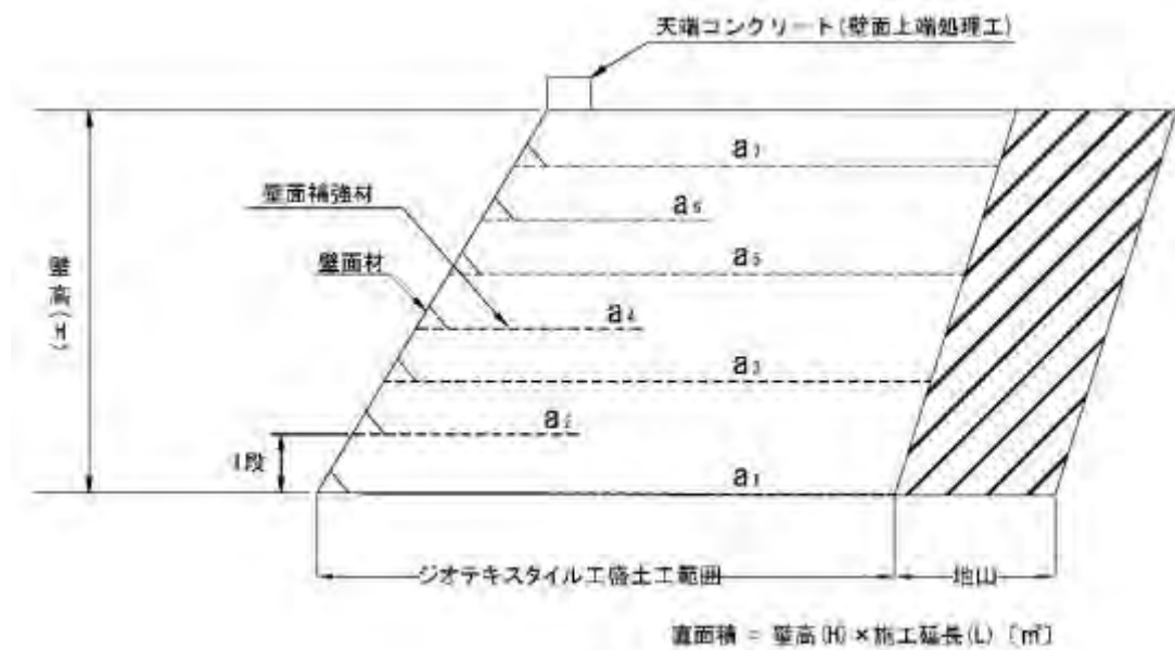
[参考図] 補強盛土工標準断面図
