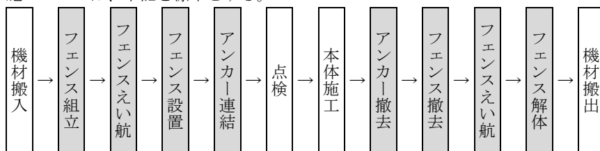
図 2-1 施工フロー
