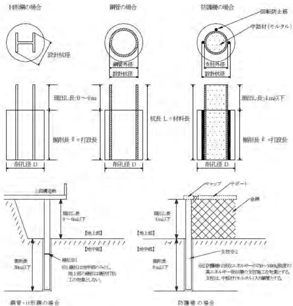
図 1-1 施工図
