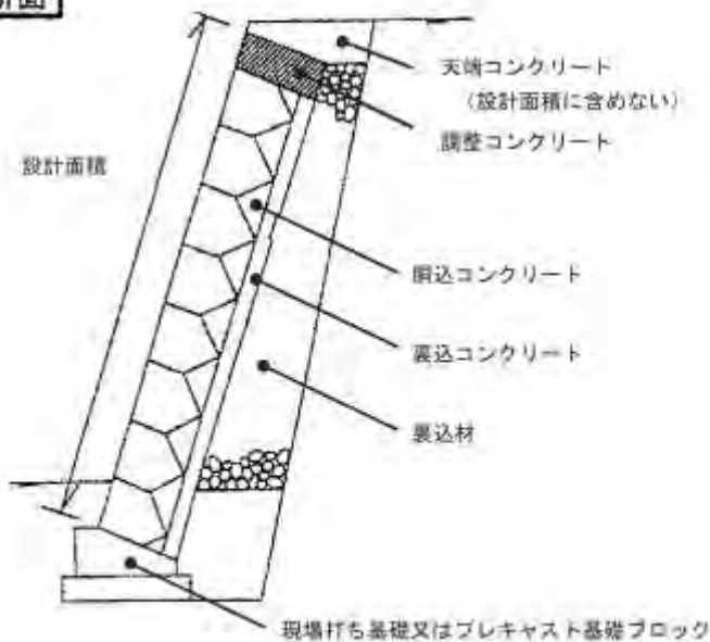
A-A断面
