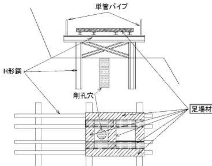
(足場概念図)
