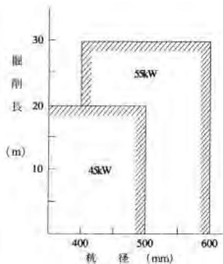
図 3-1 アースオーガの選定
