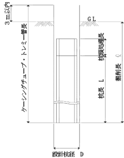
図 5-1 施工図
