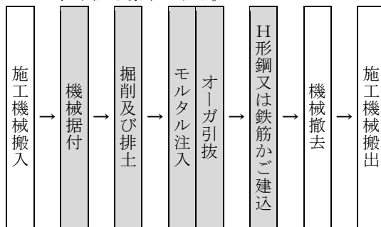
図 2-1 施工フロー
