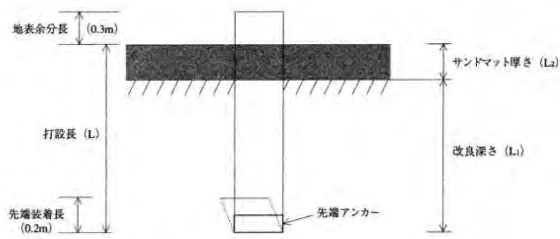
図 5.1 施工図
