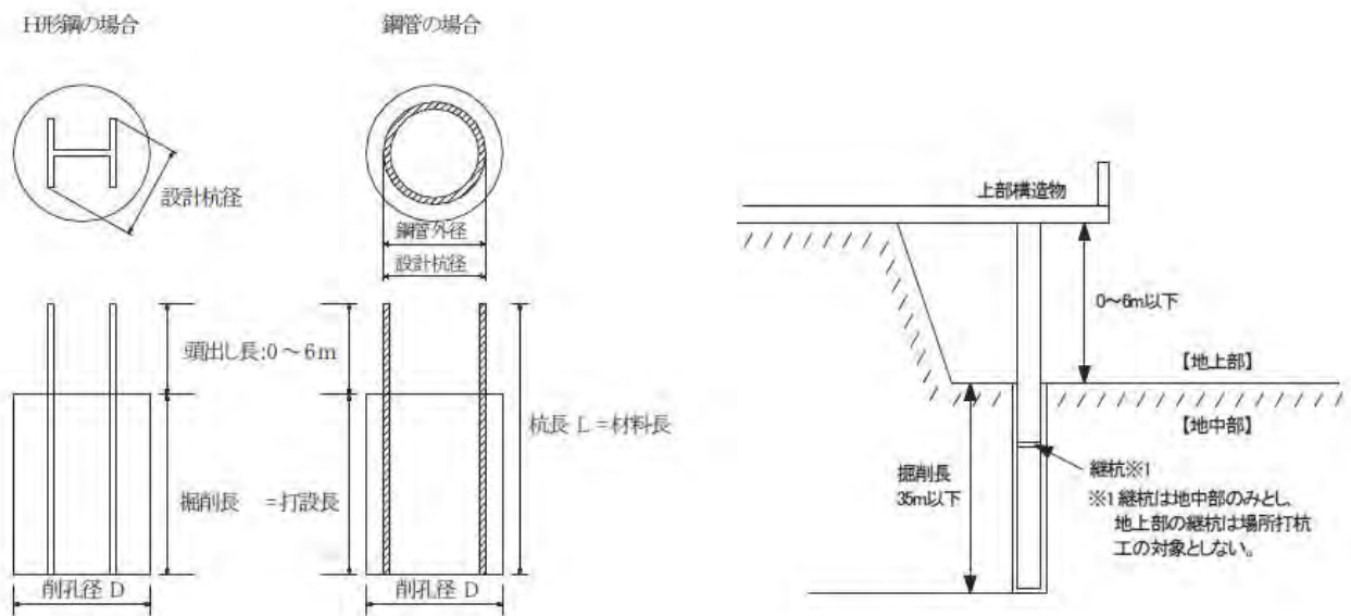
図 1-1 施工図
