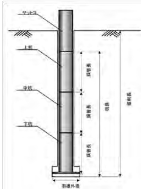
図 1-1 施工図
