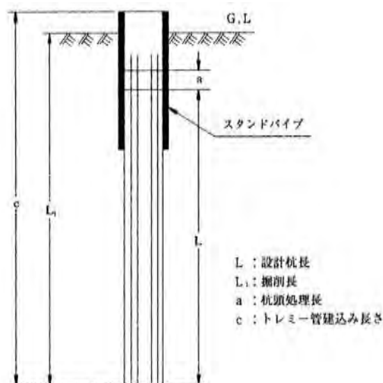
図 4-1 施工図
