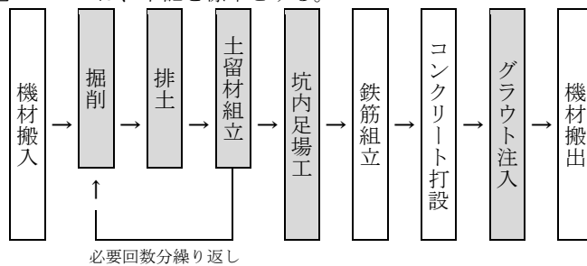
図 2-1 施工フロー
