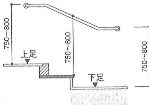
図表5-22 玄関手すり設置例
