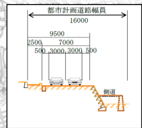
長東八木線 標準断面図
