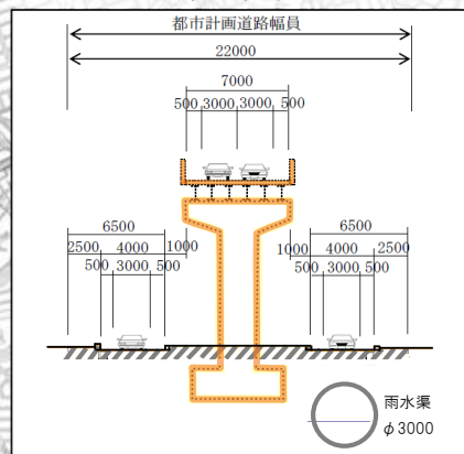
川の内線 標準断面図
