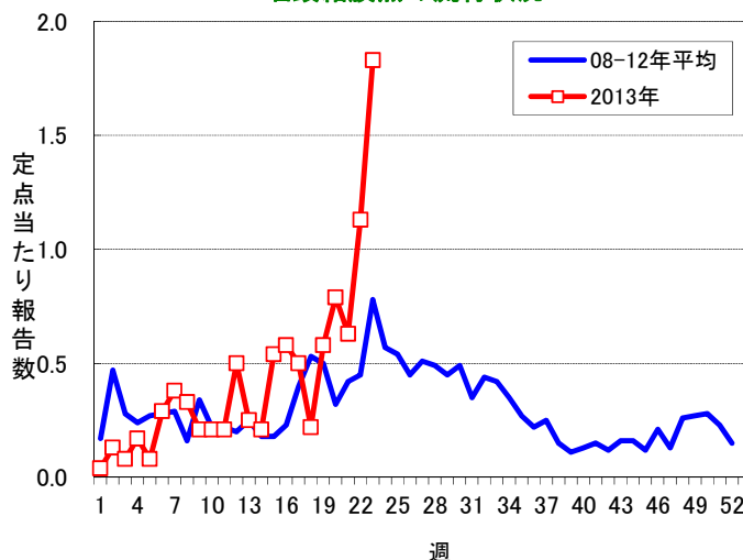
咽頭結膜熱の流行状況
