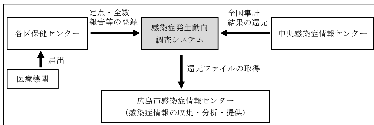
図 1 感染症発生動向調査システムによるデータ取得フロー(広島市)
