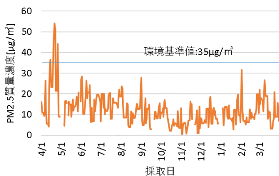
図 2-1 当所における採取日毎のPM2.5質量濃度の年間推移
