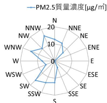
図 2-3 各風向のPM2.5平均質量濃度
