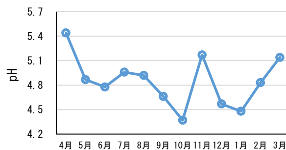
図 3 月別の pH
