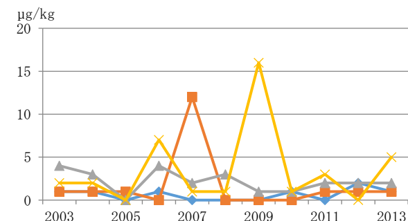
図 4 TPT の調査結果(海域・底質)
