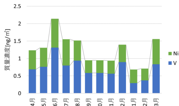
図 5-1 石油燃焼由来成分の年間推移
