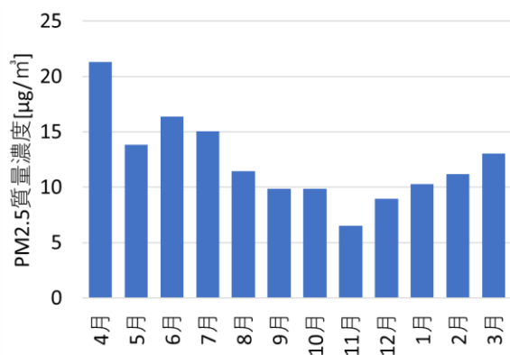
図 2-2 月平均のPM2.5質量濃度の年間推移
