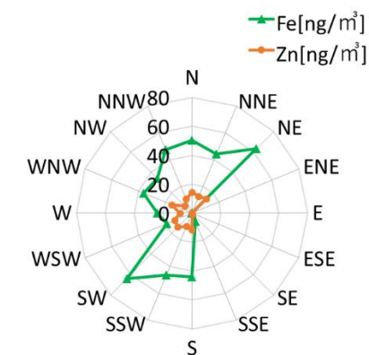
図 4-2 鉄鋼業由来成分の風向と濃度の関係
