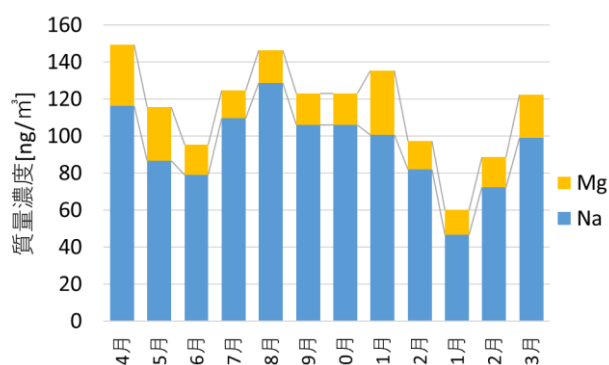
図 3-1 海塩由来成分の年間推移
