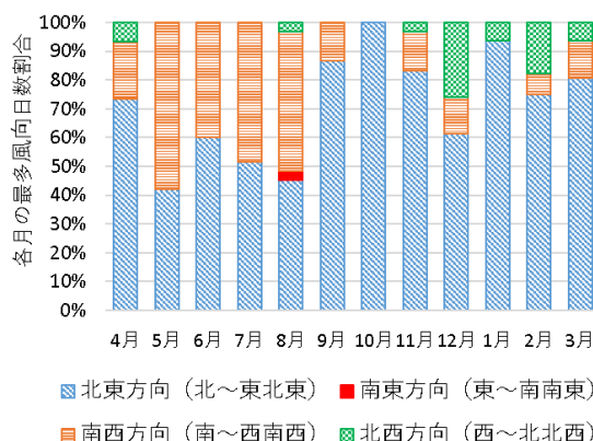
図 2-4 各月の最多風向日数の割合
