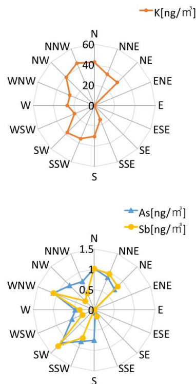
図7-2 野焼き, 廃棄物焼却由来成分の風向と濃度の関係
