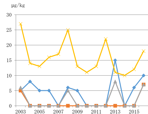
図 6 ビスフェノール A の調査結果(海域・底質)
