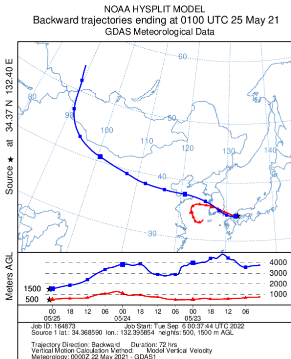
図8 5月25日の後方流跡線解析
