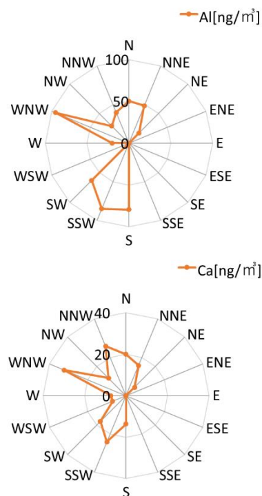
図6-2 土壌由来成分の風向と濃度の関係
