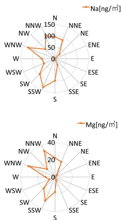
図 3-2 海塩由来成分の風向と濃度の関係
