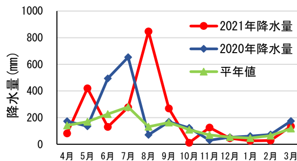
図 2 月別降水量
