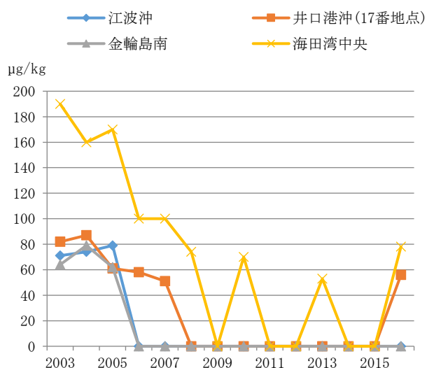
図 5 ノニルフェノールの調査結果(海域・底質)
