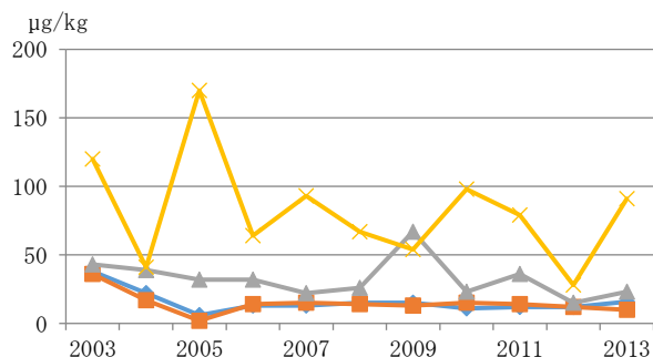
図 3 TBT の調査結果(海域・底質)
