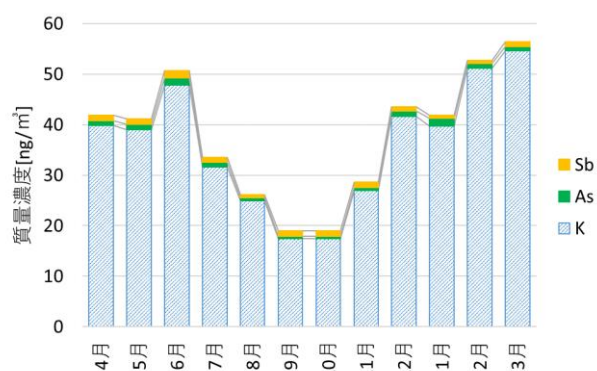
図7-1 野焼き, 廃棄物焼却由来成分の年間推移
