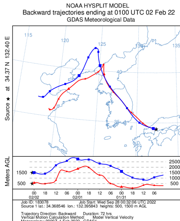
図 12 2月2日の後方流跡線解析
