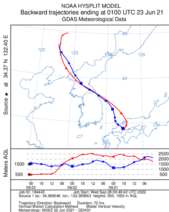
図9 6月23日の後方流跡線解析
