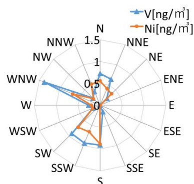
図 5-2 石油燃焼由来成分の風向と濃度の関係
