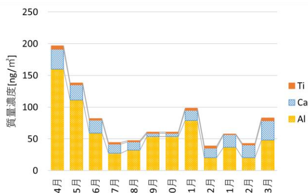
図6-1 土壌由来成分の年間推移
