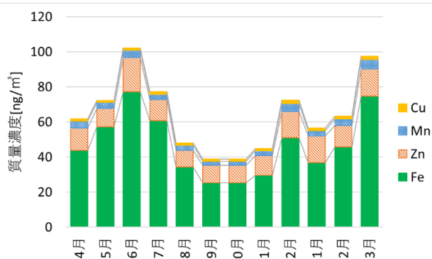
図 4-1 鉄鋼業由来成分の年間推移
