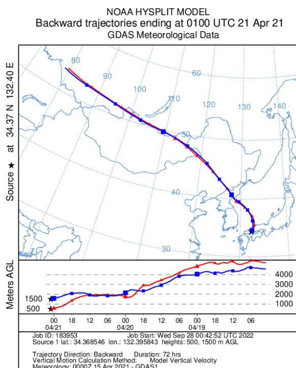
図 13 4 月 21 日の後方流跡線解析
