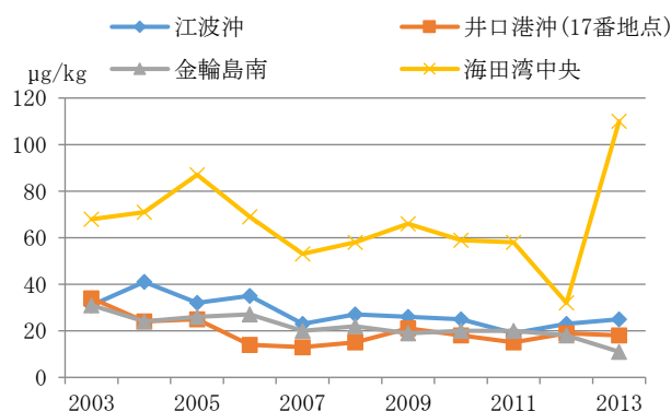
図 2 PCB の調査結果(海域・底質)
