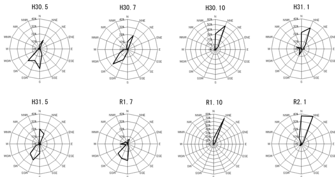
図5 各調査期間中の風配図(気象庁観測所「広島」のデータより)
