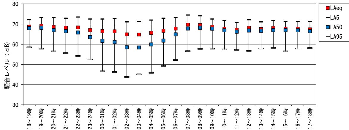
図3-4(4) 道路交通騒音の調査結果（地点：JN2、休日）
