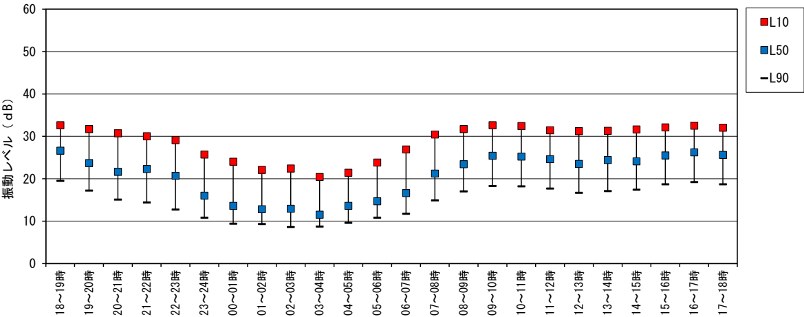
図4-4(2) 道路交通振動の調査結果（地点：JV1、休日）
