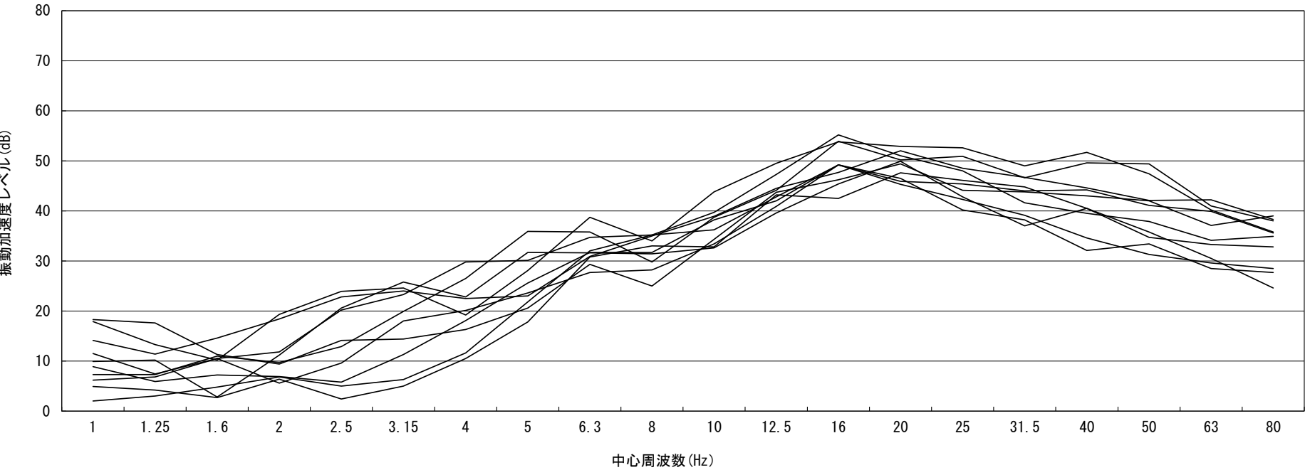
図4-5(3) 地盤卓越振動数の調査結果（地点：JV3）
