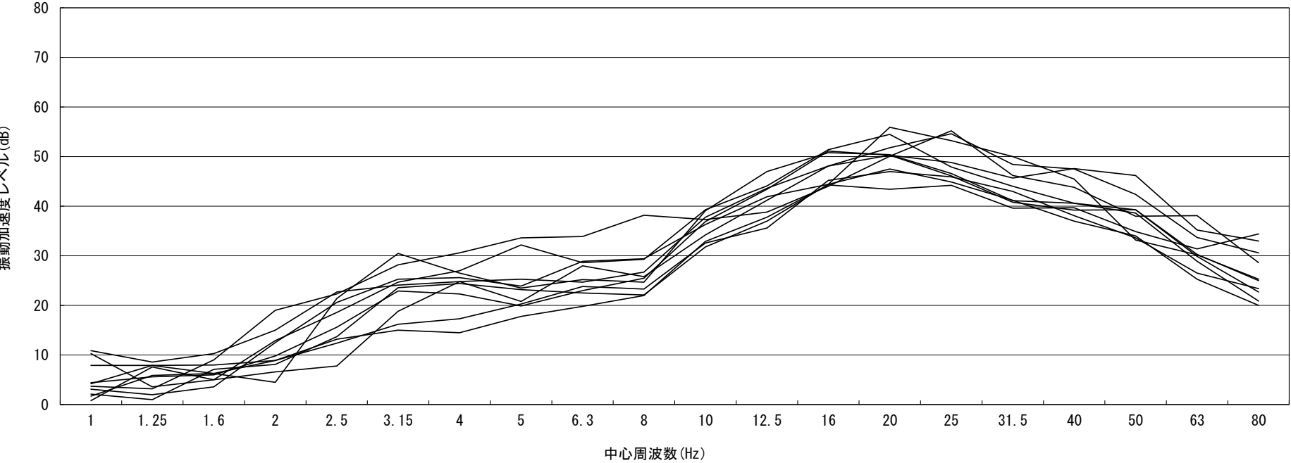
図4-5(1) 地盤卓越振動数の調査結果（地点：JV1）
