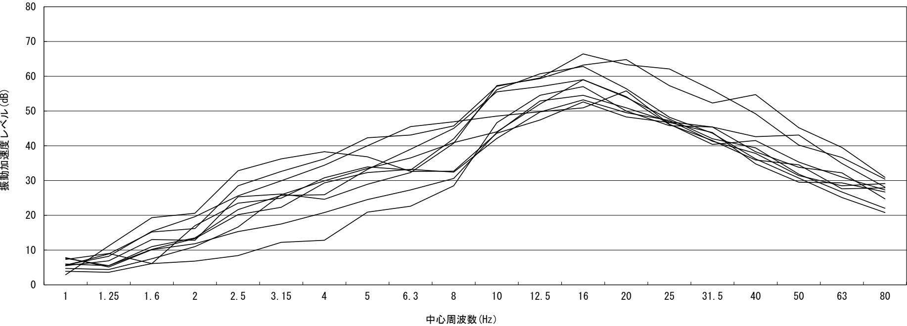
図4-5(2) 地盤卓越振動数の調査結果（地点：JV2）
