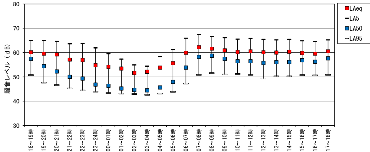
図3-4(1) 道路交通騒音の調査結果（地点：JN1、平日）
