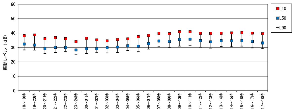
図4-3(3) 環境振動の調査結果（地点：KV2、平日）
