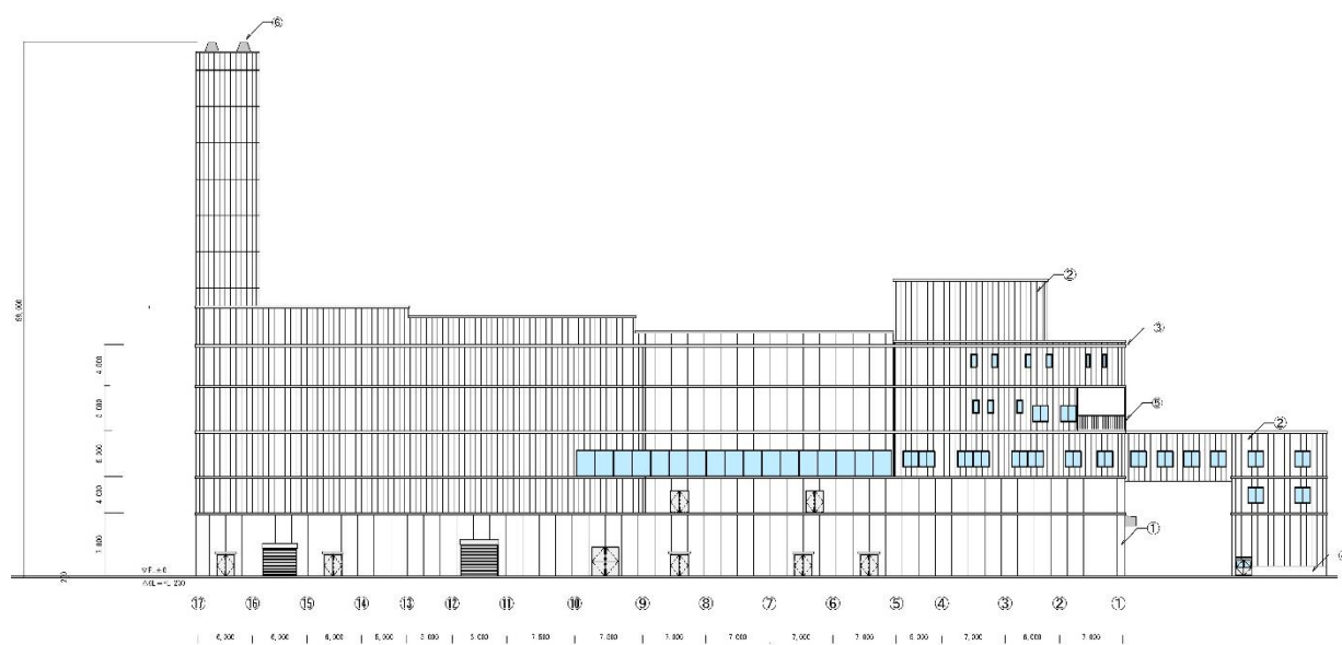
東側立面図
