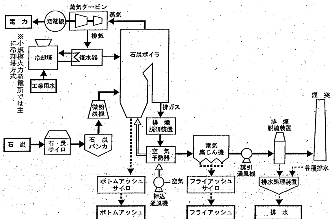
図5 小規模火力発電所における火力発電（PC・石炭）の発電設備フロー図
