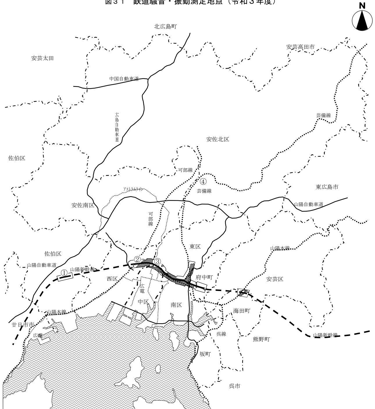
図3 1 鉄道騒音・振動測定地点（令和3年度）
