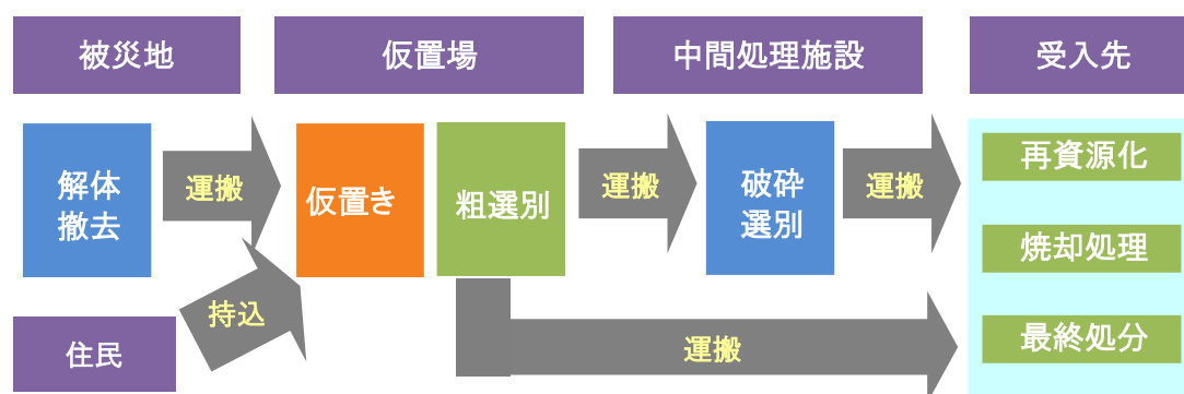
図 2-15 仮置場に搬入する災害廃棄物の処理の流れ
