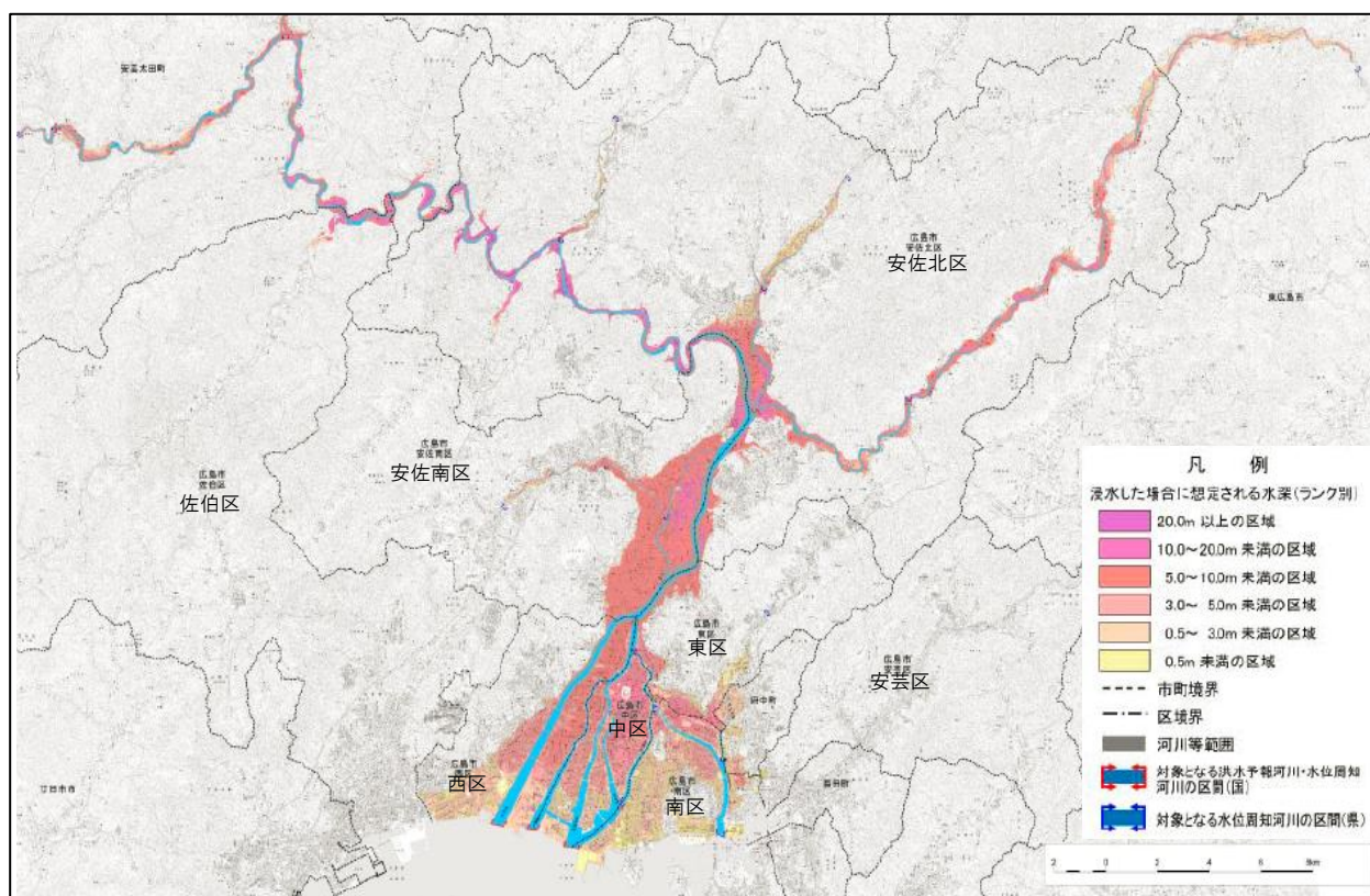
図 2-12 太田川水系洪水浸水想定区域図(想定最大規模)
