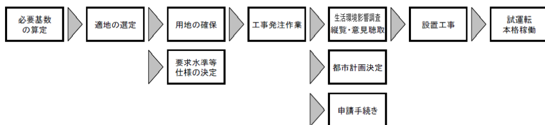
図 2-30 仮設中間処理施設（焼却施設）の設置フロー例
