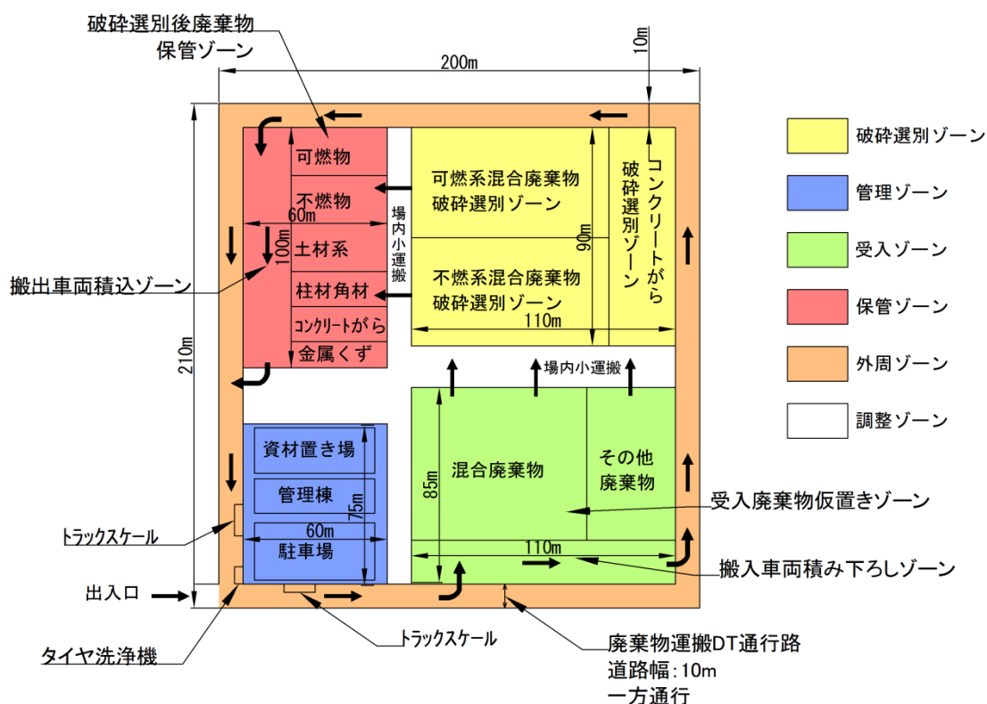
図 2-28 中間処理施設のゾーン区分と施設構成例
