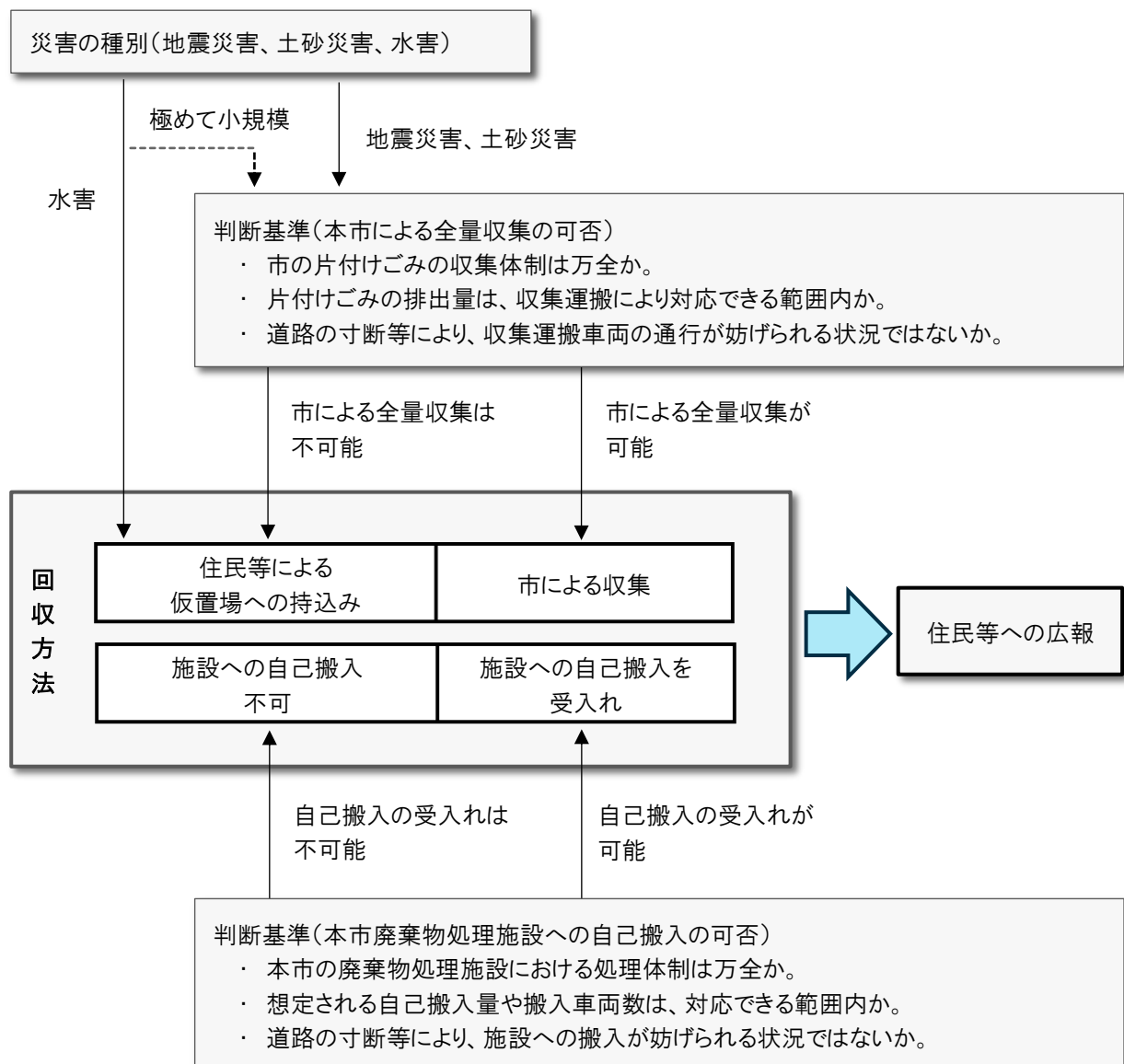
図 2-22 片付けごみの回収方法の検討フロー
