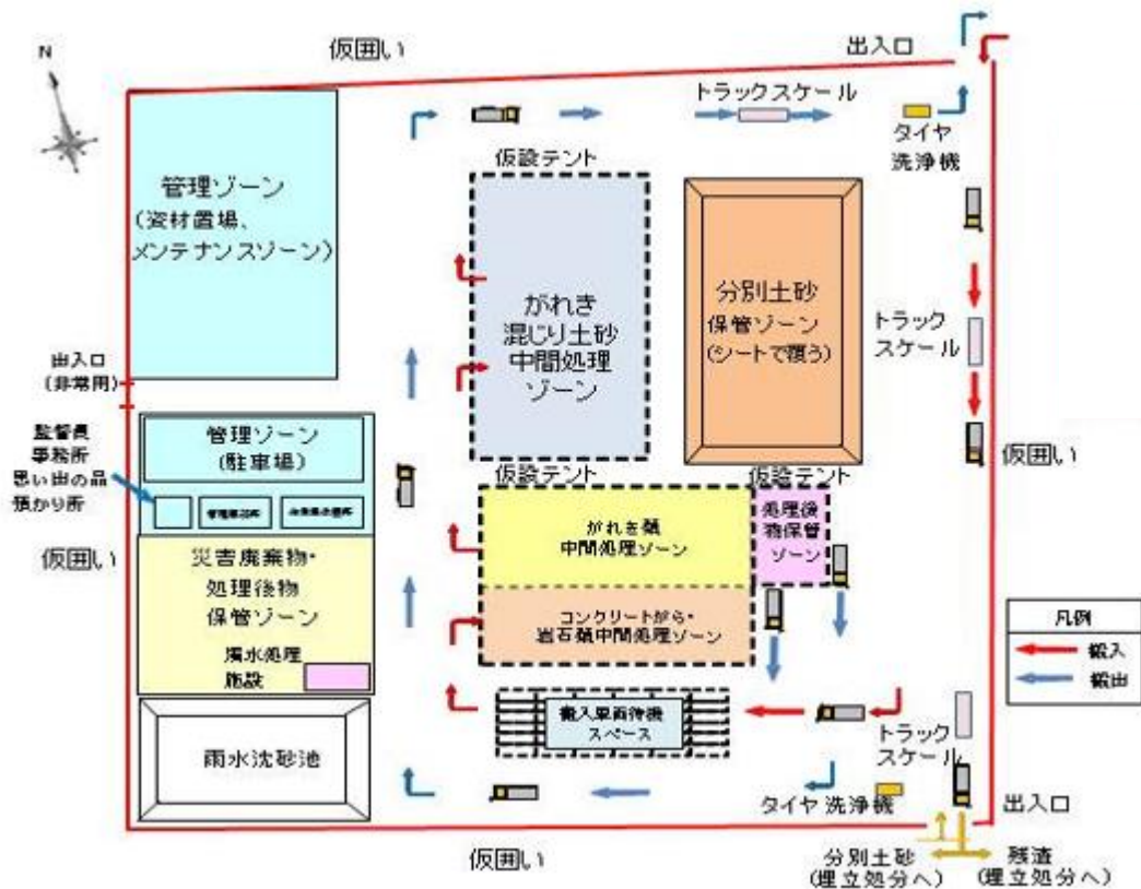
図 2-29 平成26年8月豪雨災害の際に設置した中間処理施設のレイアウト
