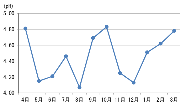
図 3 月別の pH
