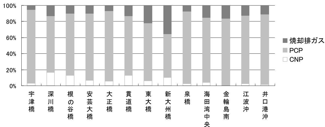
図 8 地点ごとの寄与率(PCDDs 及び PCDFs)
