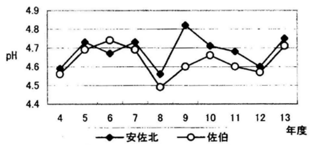
図2 pHの経年変化
