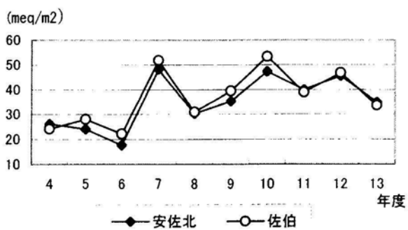
図6 NH 4 + 沈着量の経年変化
