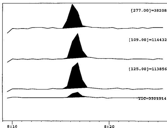
図5 フェニトロチオン 0.1mg/ℓ、2μℓ注入のMC
