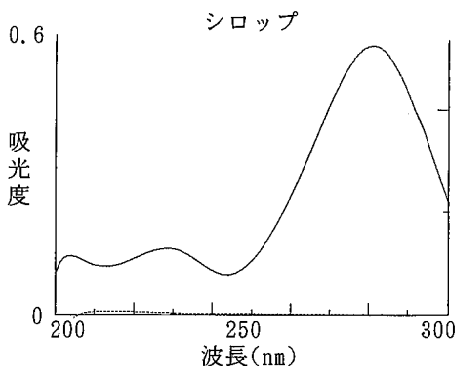
図8 実試料の試料液と固相抽出液の UV スペクトル (分析方法: BA)
