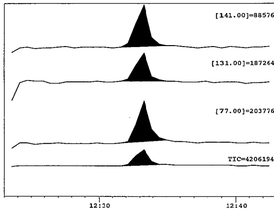
図6 ペンシクロン 0.5mg/ℓ、2μℓ注入のMC
