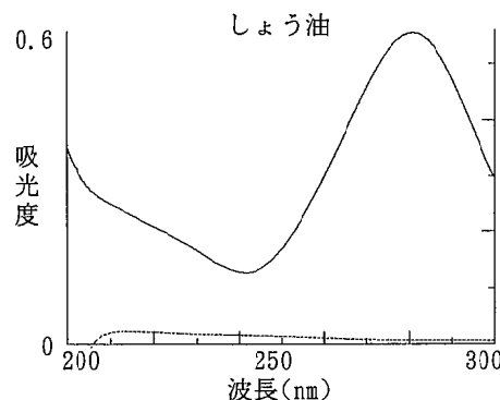
図9 実試料の試料液と固相抽出液の UV スペクトル (分析方法: PHBA-Es)
