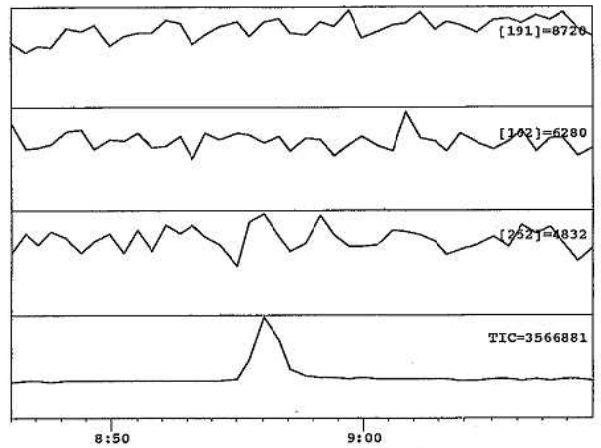
ベンディメタリンのモニターイオンで測定したキャプトラン単品のMC (1mg/ℓ, 2μℓ注入)
