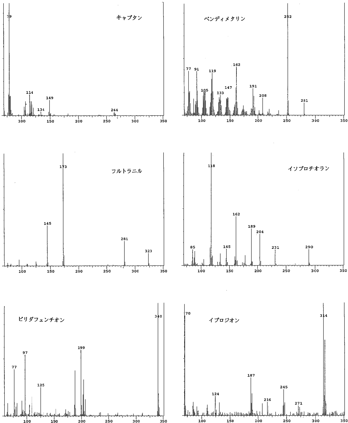
図2 重複ピークにおける単品のマスペクトル
