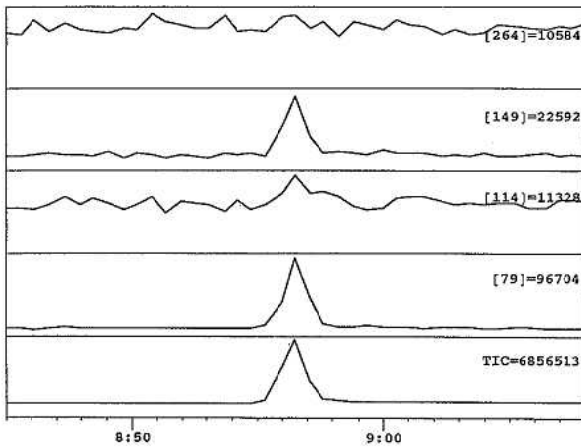
キャプトランのモニターイオンで測定したベンディメタリン単品のMC (1mg/ℓ, 2μℓ注入)
