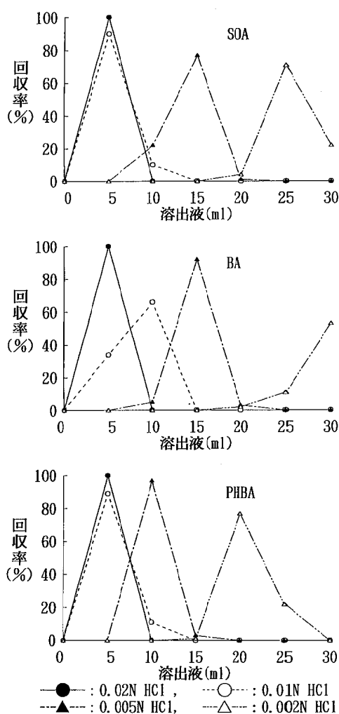
図2 SOA、BA、PHBAのSAXカラムからの溶出パターン
