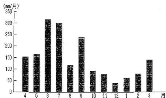
図4 月別降雨量
