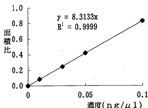
図2 t-BPhの検量線
