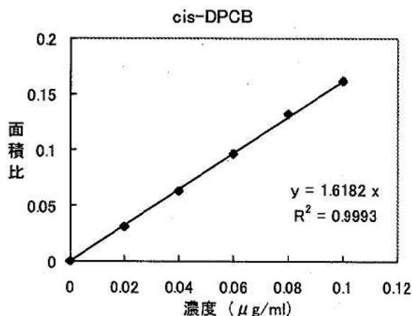
図2-1 検量線その1
