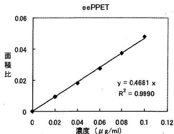
図2-2 検量線その2
