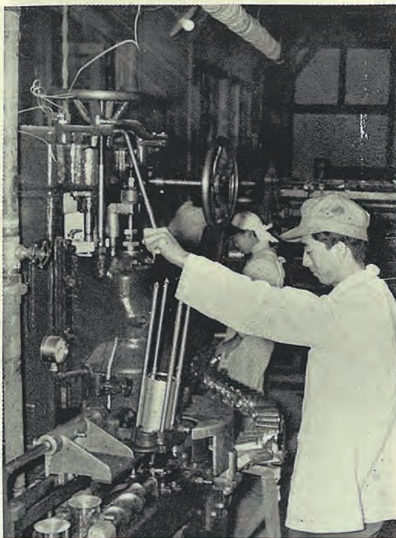
伍 詰 真空巻縮機による密閉作業
