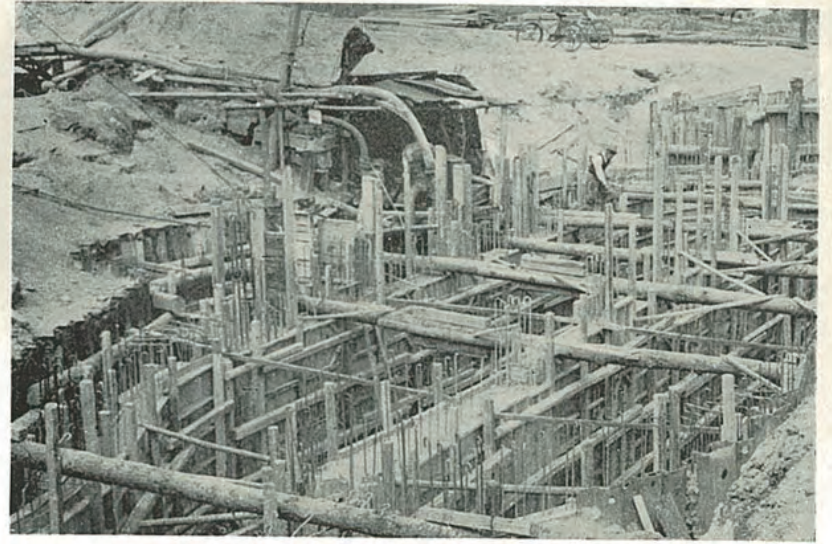
下水管埋設工事
