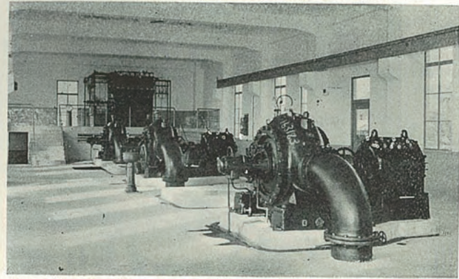
送 水 ポ ン プ
