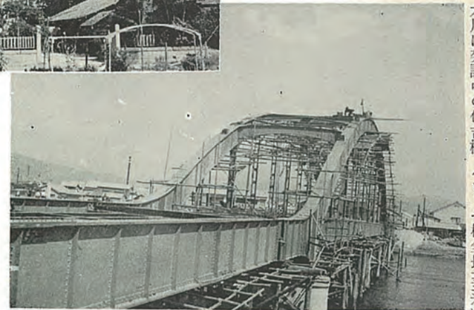
本川に架設中の住吉橋（ローゼ桁全長二三米）
