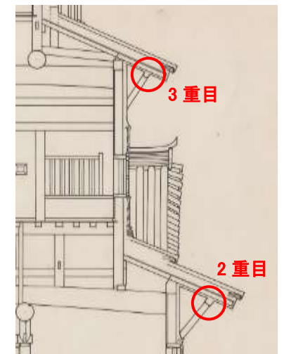
天守南北断面図(部分) 奈良文化財研究所所蔵
