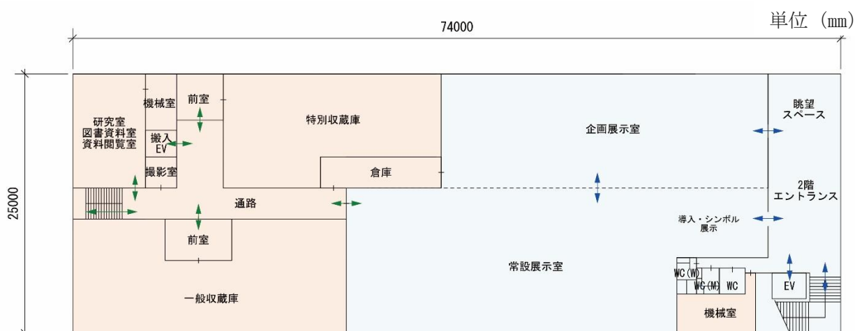
2階平面図
