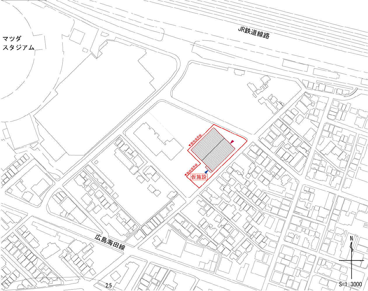
仮施設配置図
