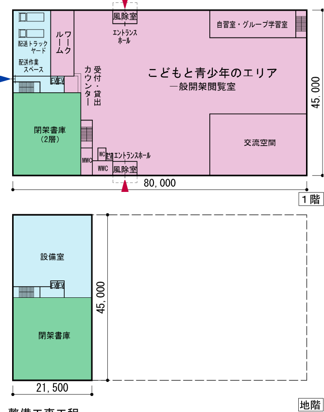
本施設平面図
