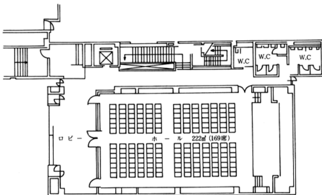
2 階 (373.95 m²)
