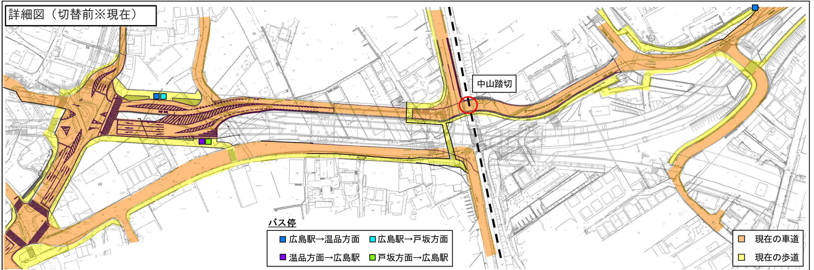
詳細図（切替後）※令和6年度末までの道路形態（予定）
