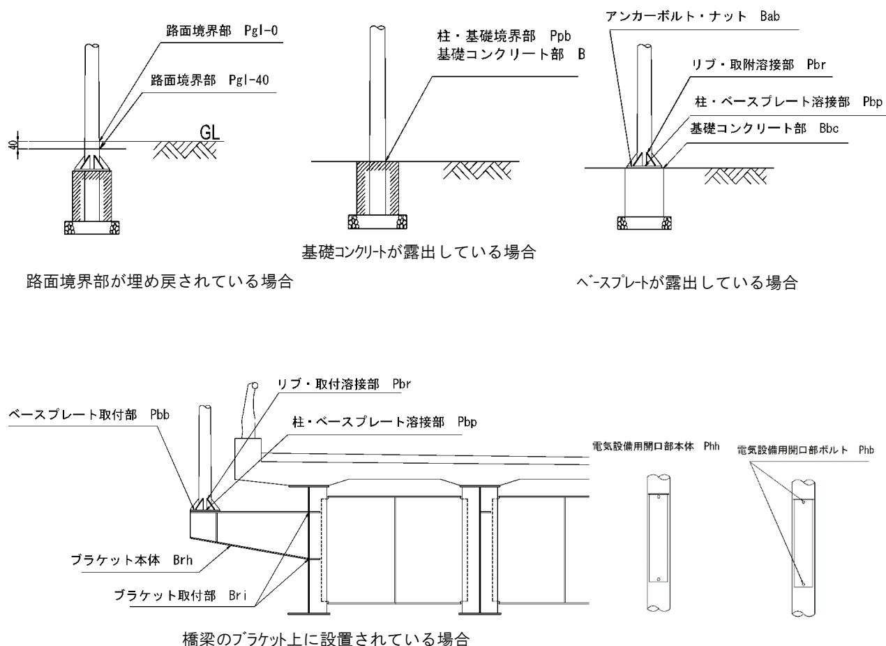
図 8-3 主な点検箇所（支柱基部および電気設備用開口部）
