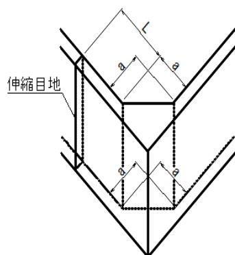
(立面図)
