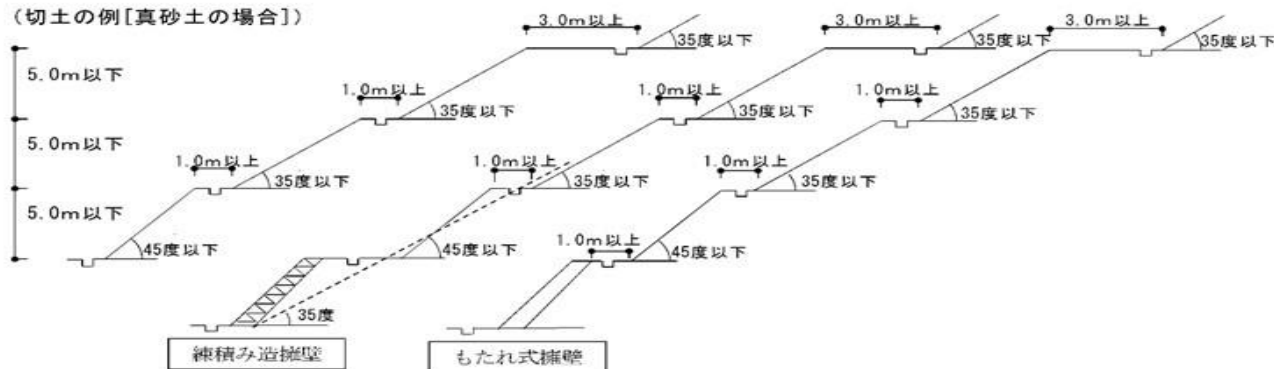
(盛土の例)
