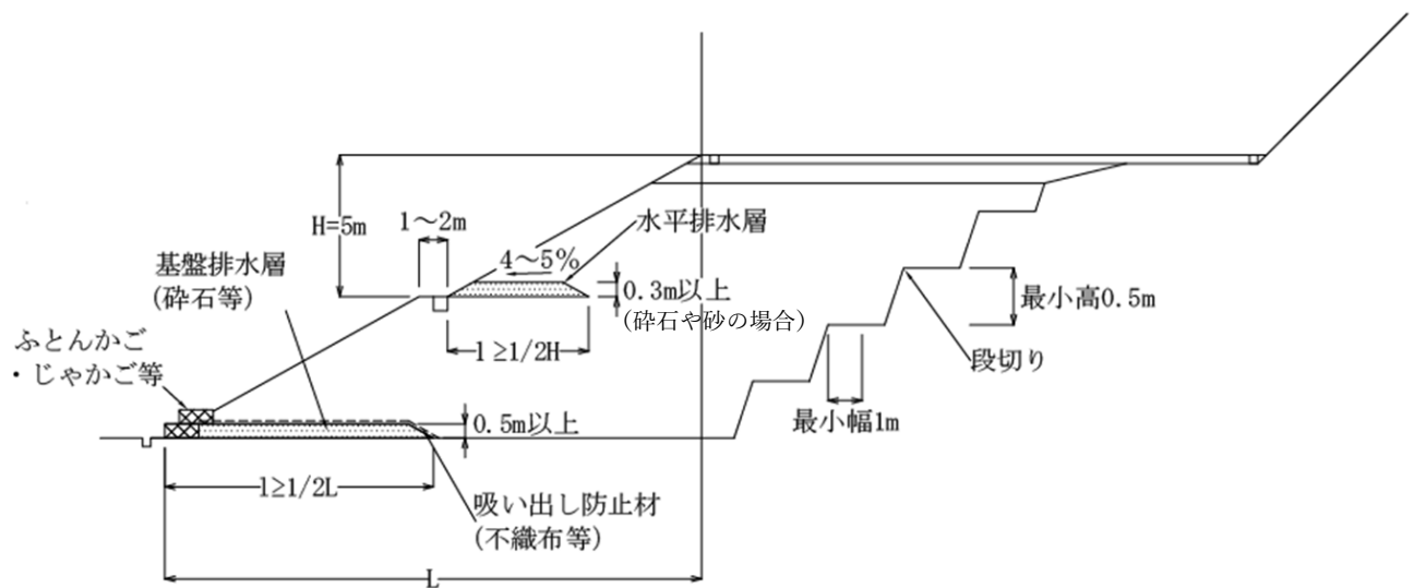
【断面図】
