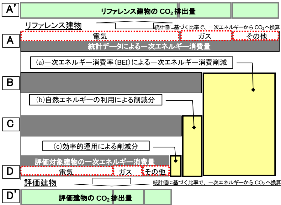
図Ⅲ. 5 評価対象建物の CO 2 排出量算定の考え方
