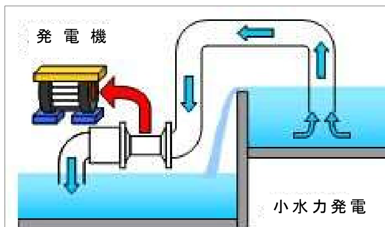
図－21 下水道施設（処理場）内の落差を利用した小水力発電の例（イメージ）
