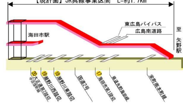
【現計画】JR呉線事業区間 L=約1.7km
