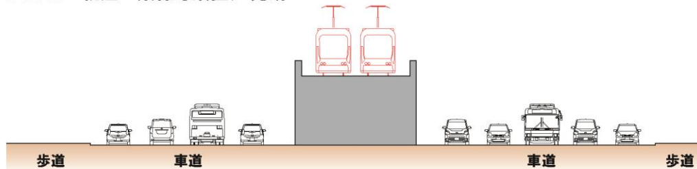
図 2-6(2) 施行順序図（高架部：軽量盛土）
