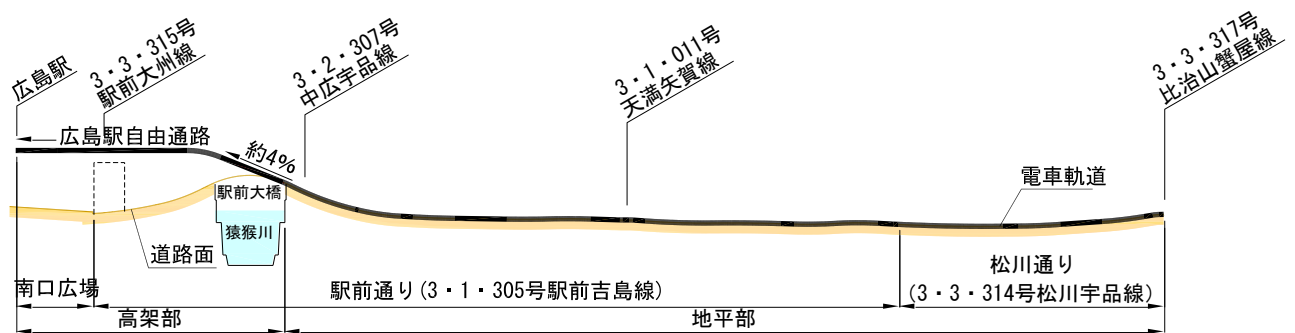
図 2-3(1) 計画縦断面図
