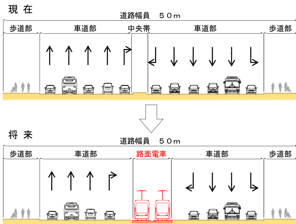
図 2-4(2) 計画横断図（地平部：B－B' 断面）
