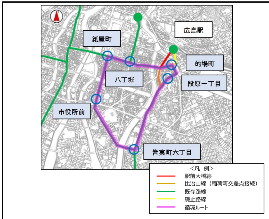
図 2-12 循環ルート図
