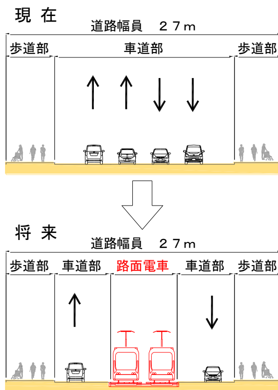
図 2-4(3) 計画横断図（地平部：C－C' 断面）
