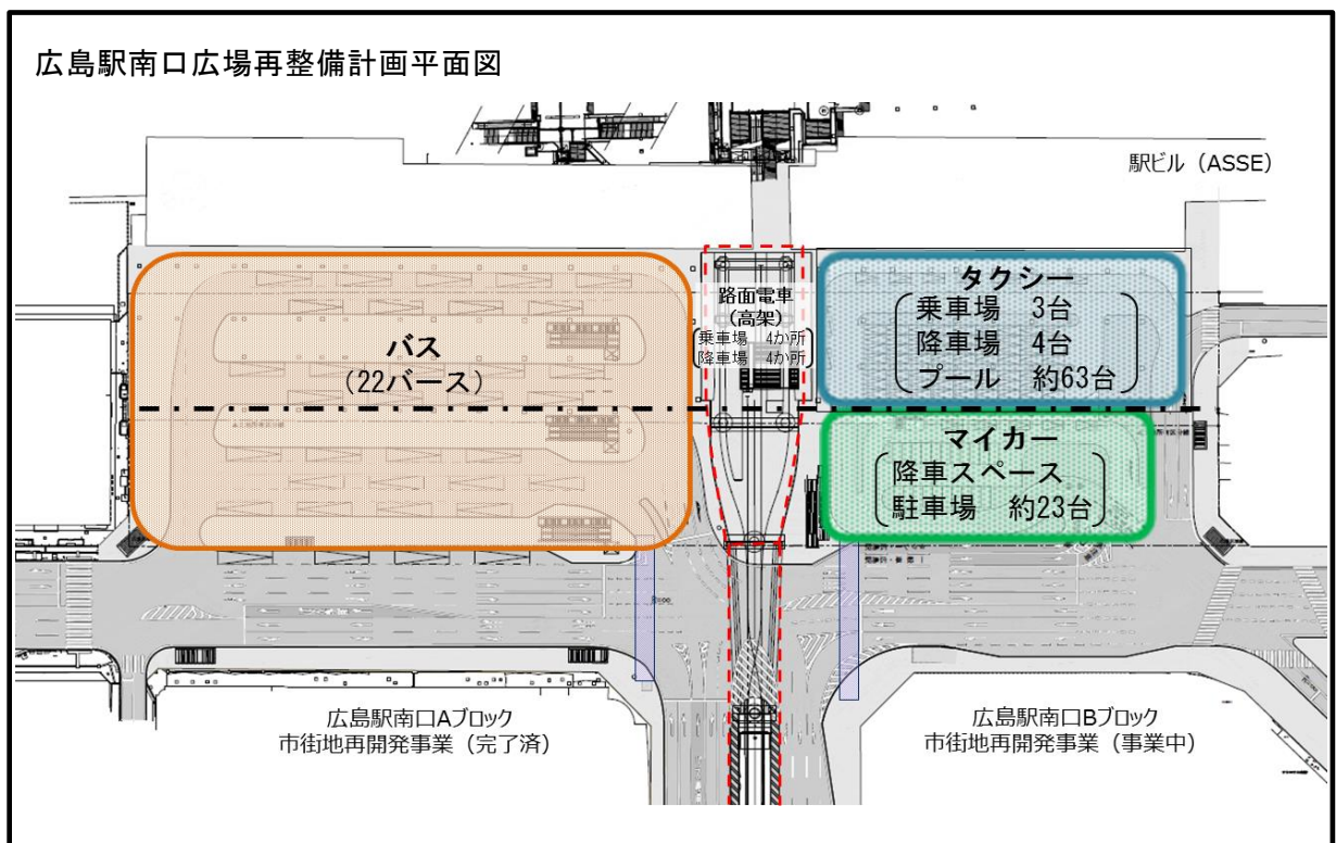
図 2-11 広島駅南口広場再整備等事業の計画概要図
