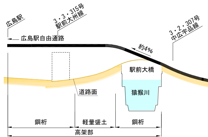
図 2-3(2) 計画縦断面図（高架部拡大）
