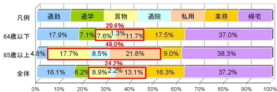
図-2 年齢階層別の移動目的（平成 20 年）
