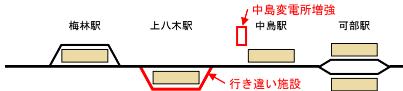
図-47 配線略図
