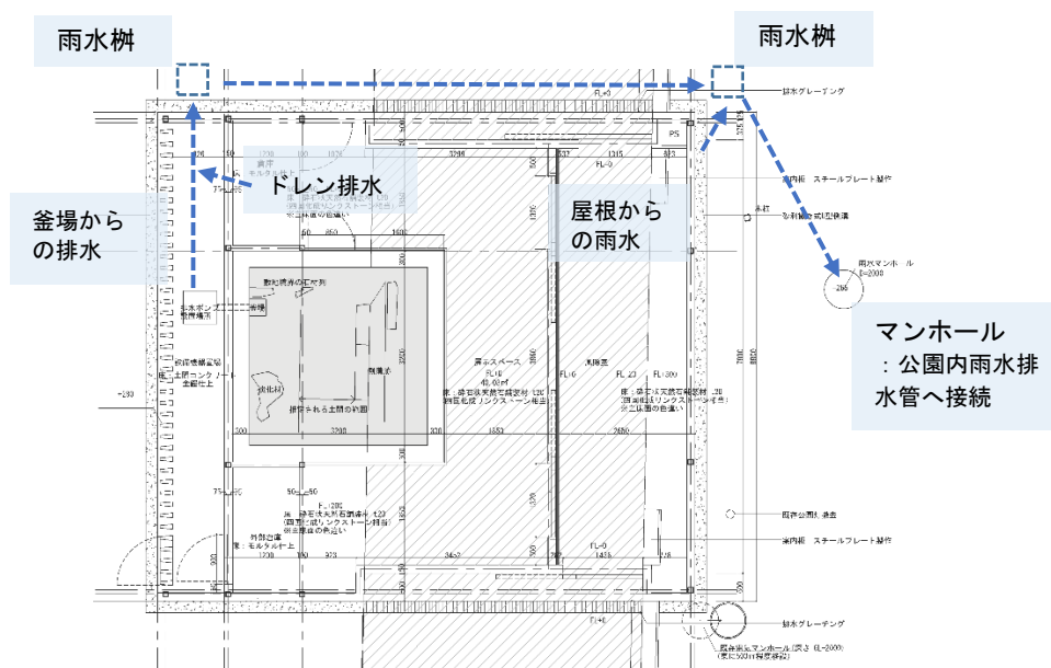
図 2.6-2 平面図
