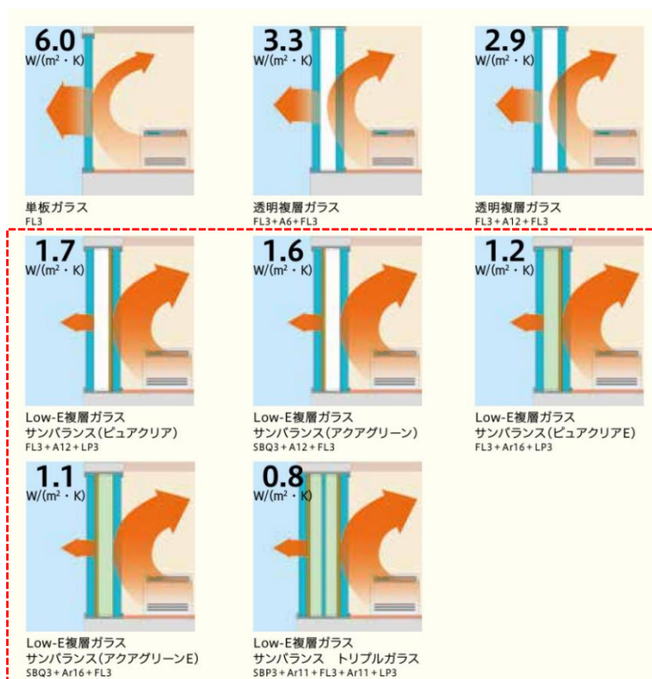
図 2.4-5 ガラスの断熱性能（出典：旭硝子）
