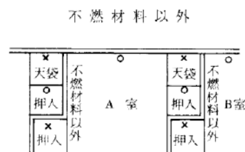
1 箇所の押入等をそれぞれA室とB室で使用している場合で押入等の壁面及び天井面が不燃材料以外のもの
