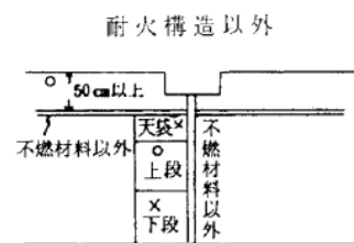
天井裏に感知器がある場合で押入等の壁面が不燃材料以外のもの
