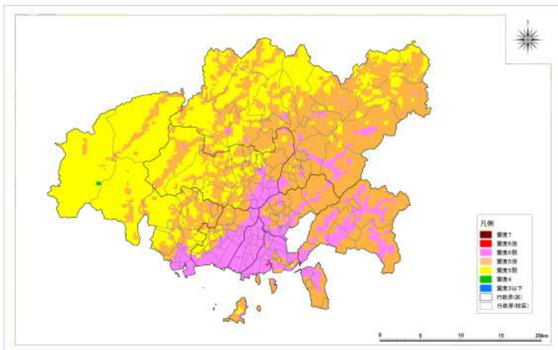
図 I 4.1(1) 震度分布図
