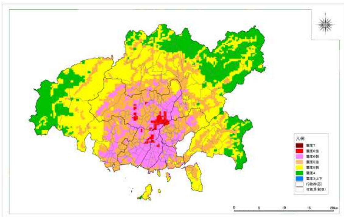
図 I 4.1(2) 震度分布図
