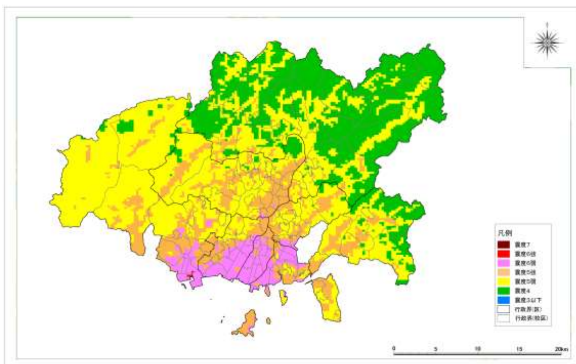
図 I 4.1(3) 震度分布図
