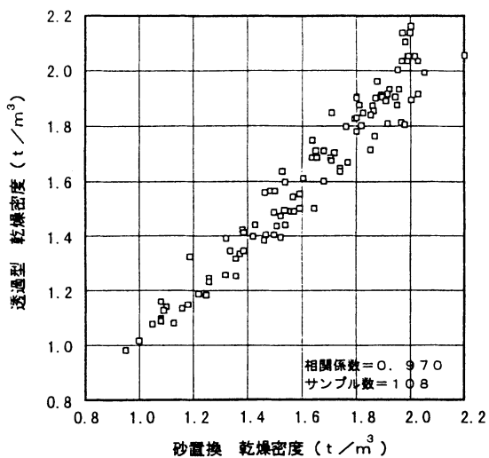
図一 5 砂置換と透過型の相関（乾燥密度・全データ）
