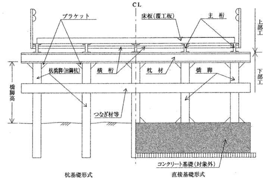
図 2-2 仮橋・仮栈橋工概念図
