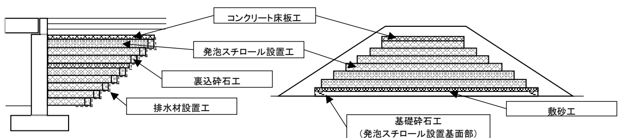
橋台裏込
