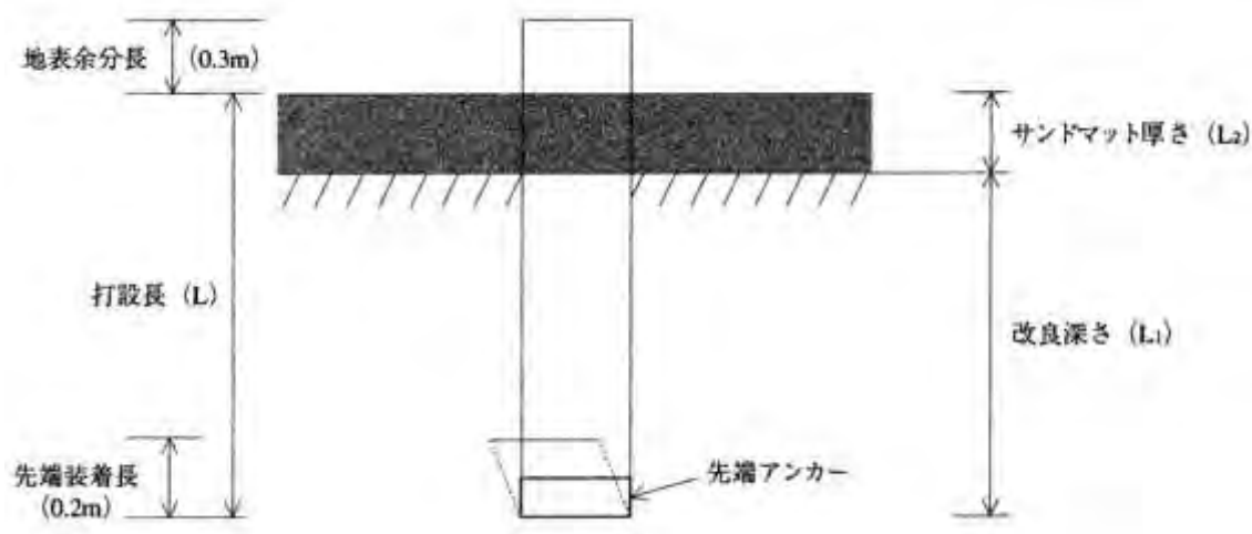
図 5.1 施工図
