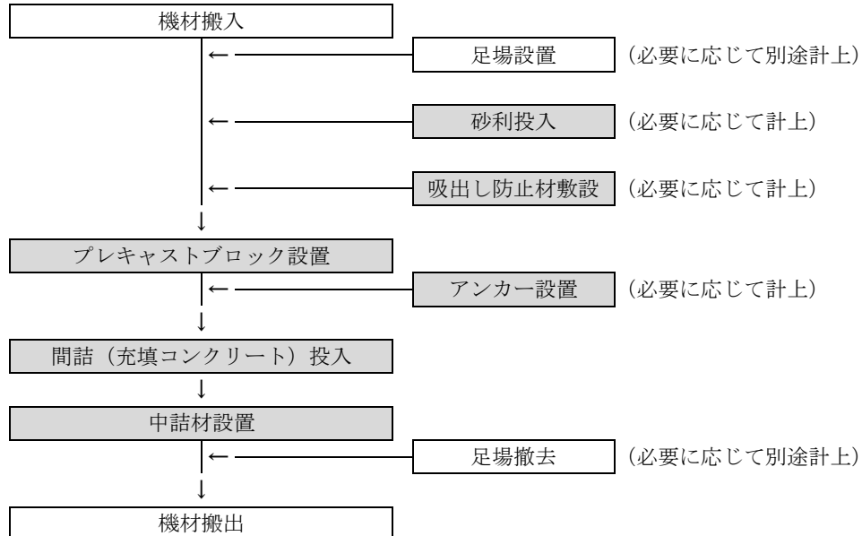
図 1-1 施工フロー
