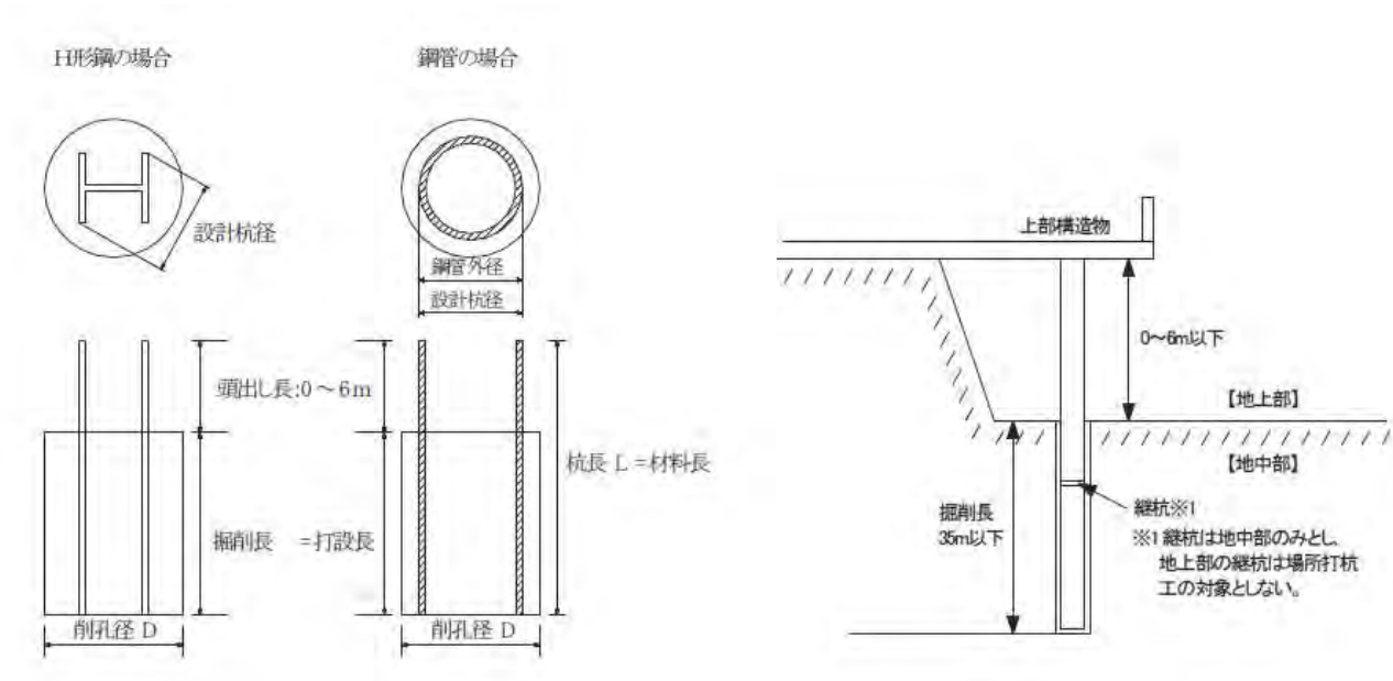
図 1-1 施工図
