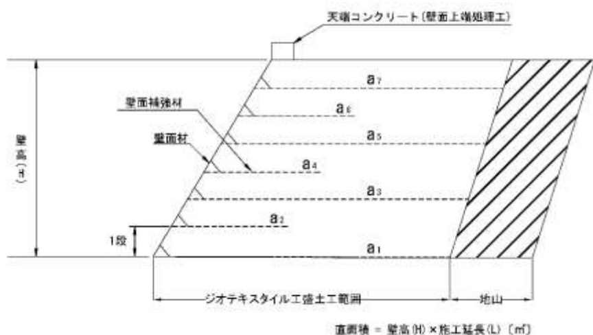
図 3.1 補強盛土工標準断面図（参考図）
