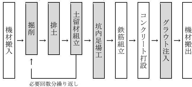
図 2-1 施工フロー
