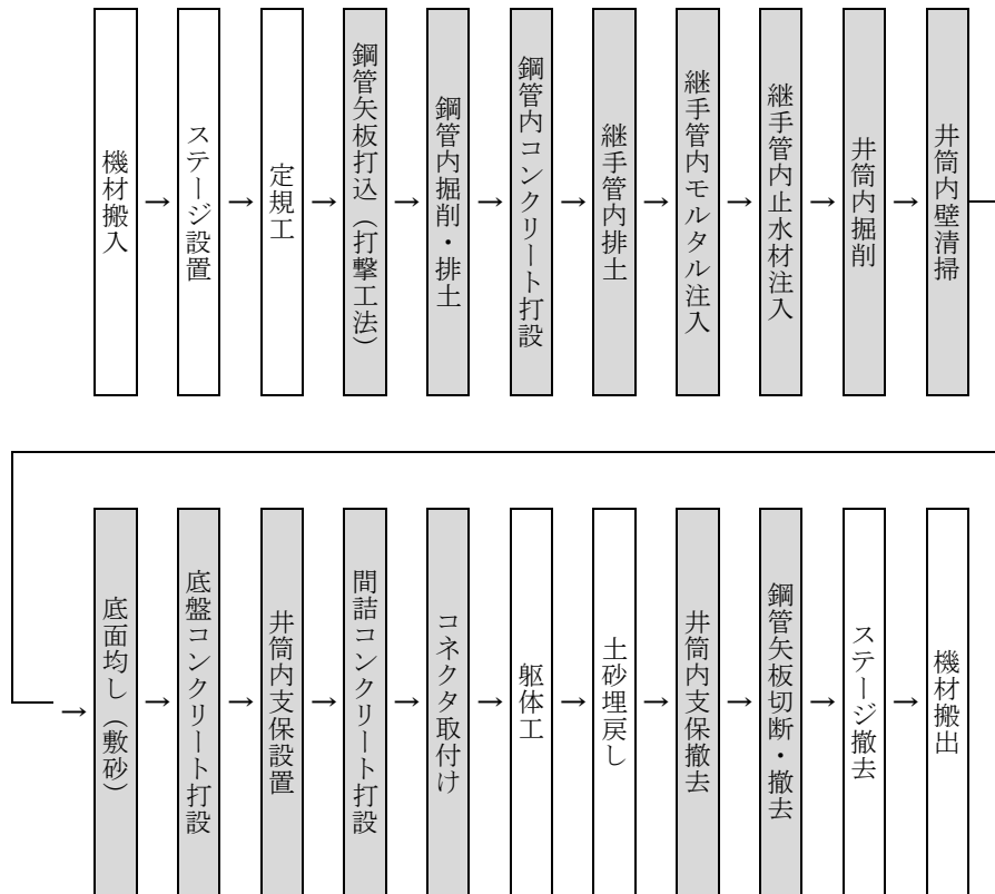
図 2-1 施工フロー
