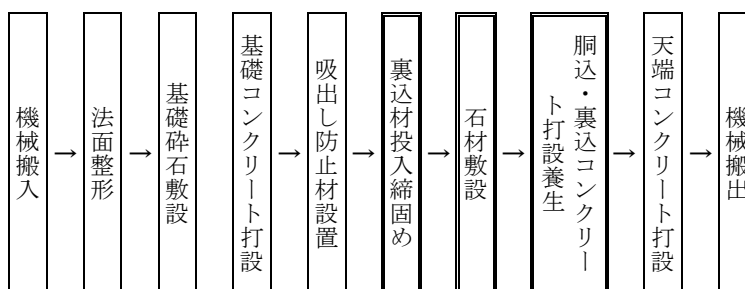
図 2-1 施工フロー
