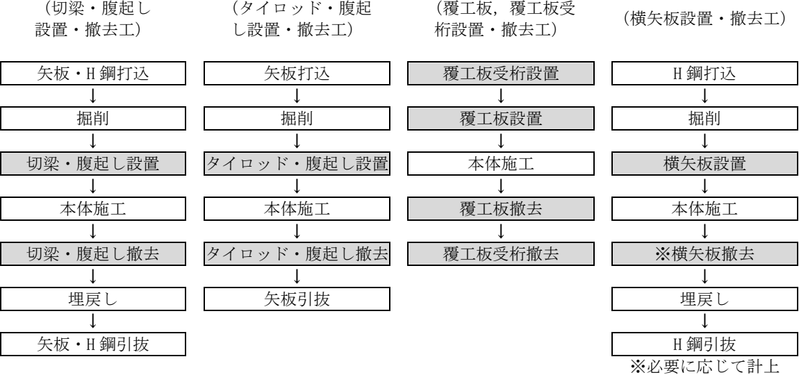
図 2-1 施工フロー
