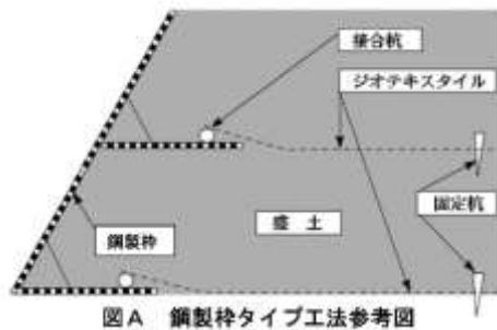
図 A 鋼製枠タイプ工法参考図
