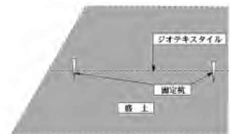
図 C 普通敷設工法（壁面材なし）参考図
