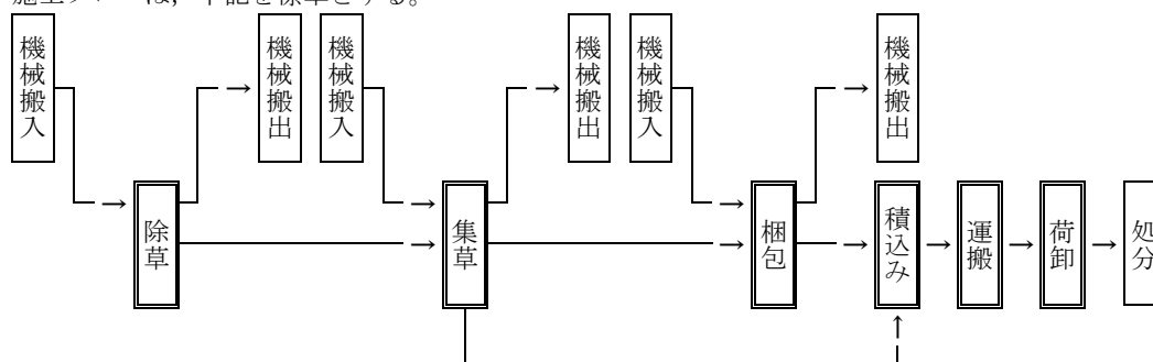
図 2-1 施工フロー
