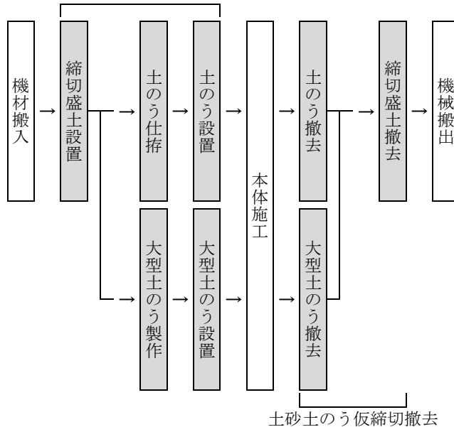
図 2.2 施工フロー
