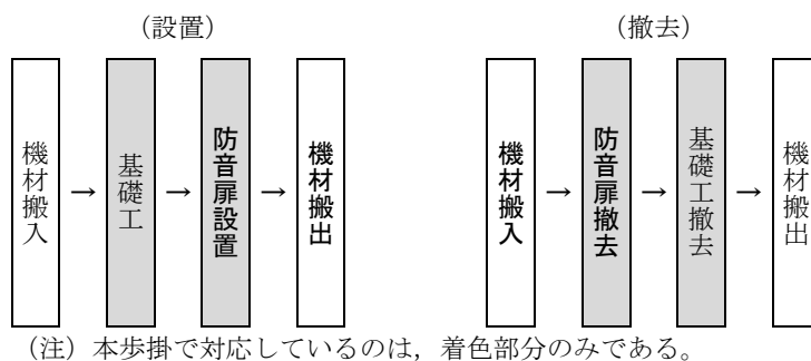
図 2-1 施工フロー
