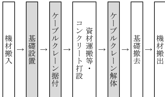
図 1-1 施工フロー
