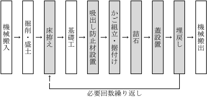
図 2-1 施工フロー
