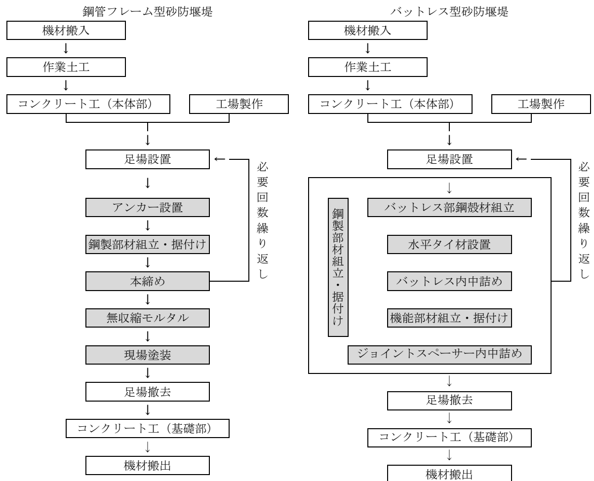
図 2-1 施工フロー
