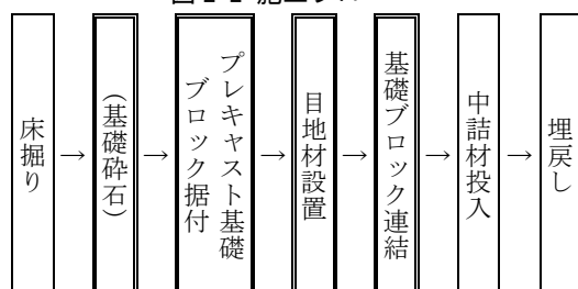
図 2-2 施工フロー
