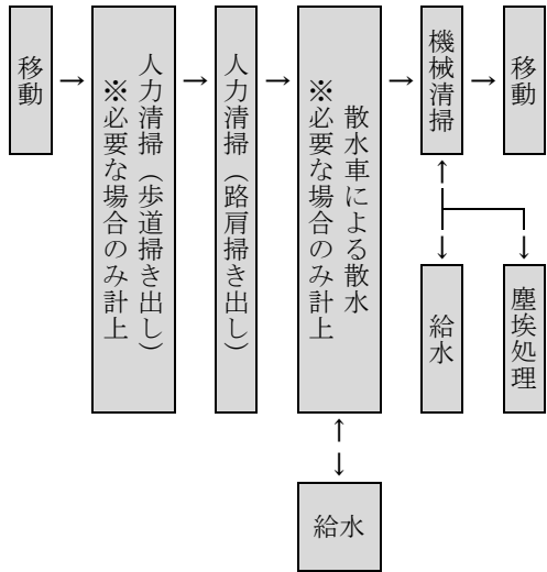
図 2-1 施工フロー
