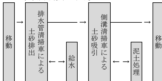
図 2-1 施工フロー
