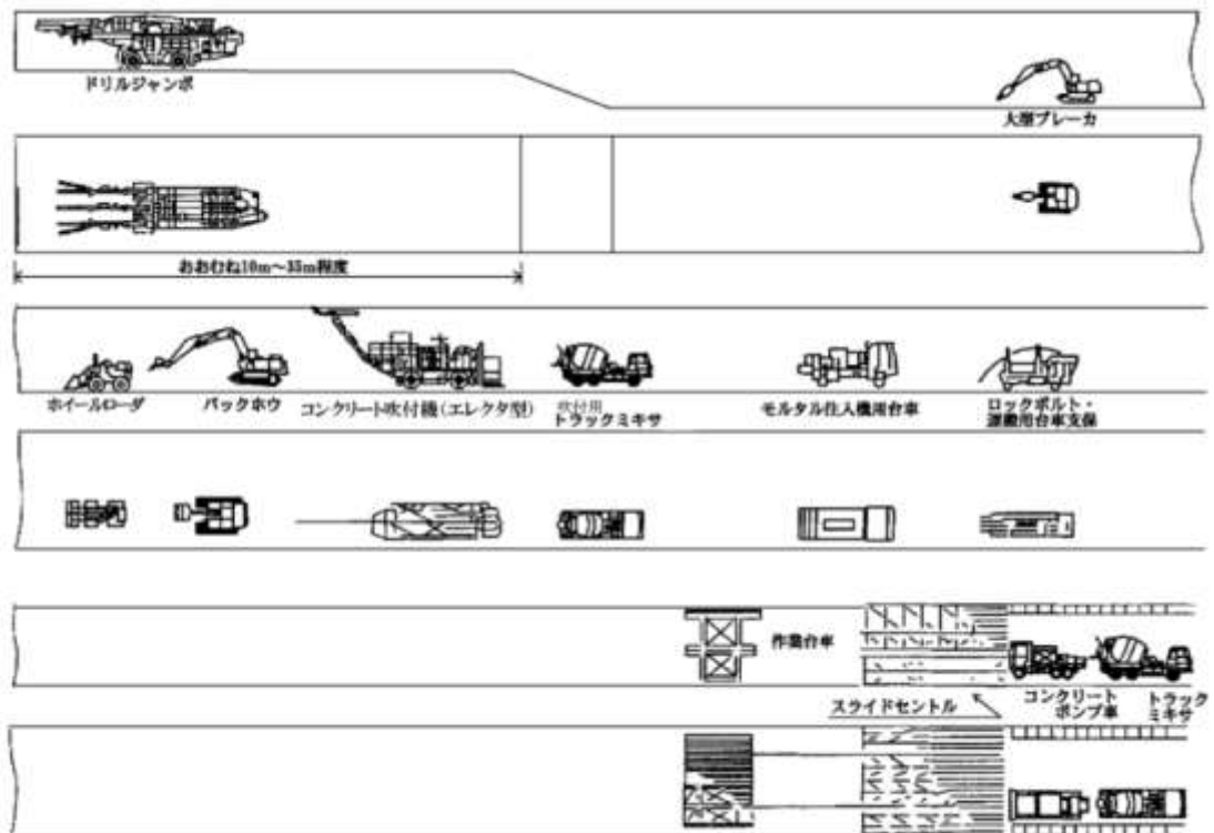
図 3.9 上半先進ベンチカット工法（上下半交互併進工法）
