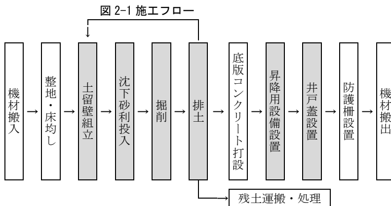
図 2-1 施工フロー
