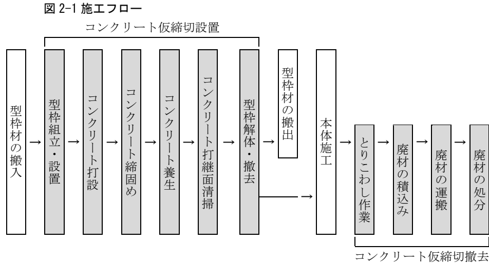
図 2-1 施工フロー
