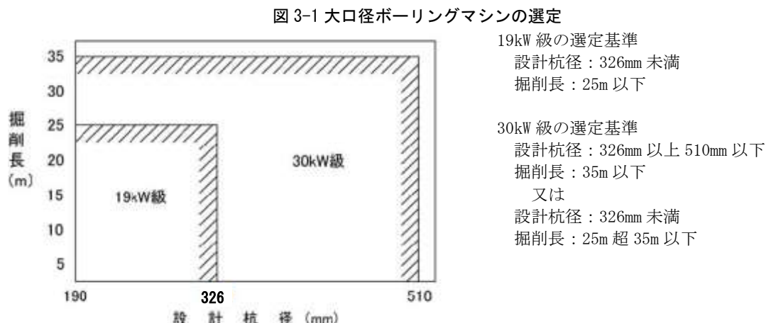
図 3-1 大口径ボーリングマシンの選定
