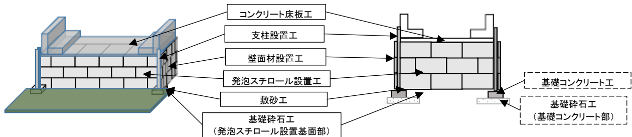
両側壁図
