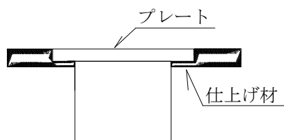
屋内運動場に使用する角型のフロアプレートの場合
