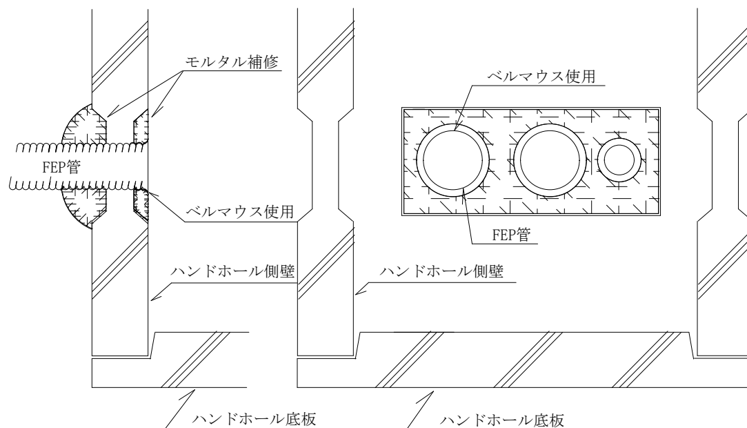
断 面 図
