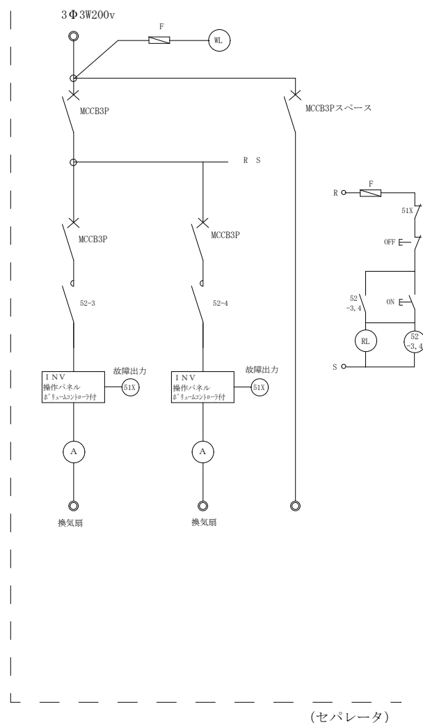
(セパレータ)
