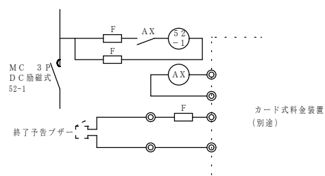
カード式料金装置回路
