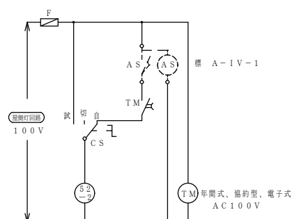
屋側灯制御回路
