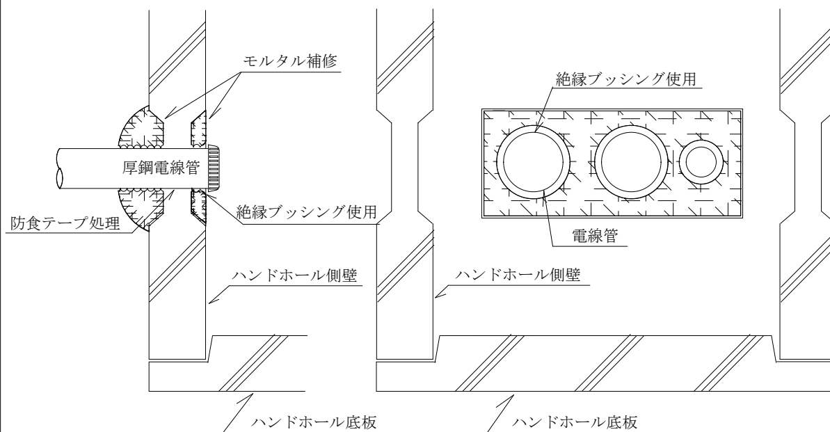
断 面 図
