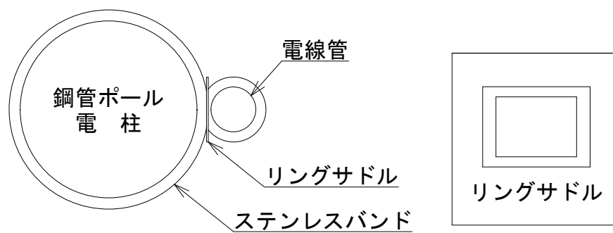
配管支持材詳細図
