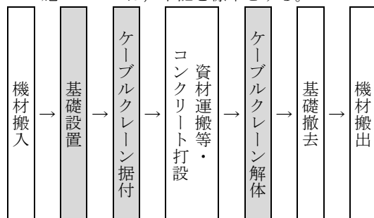
図 1-1 施工フロー
