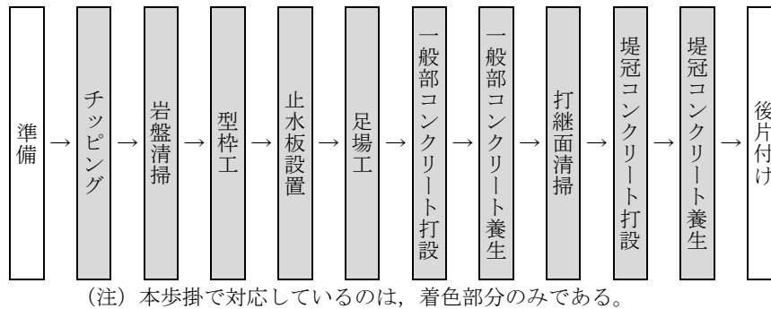
図 2-1 施工フロー
