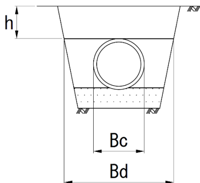
(a) 溝が広い場合 ( Bd \geq 2Bc )
