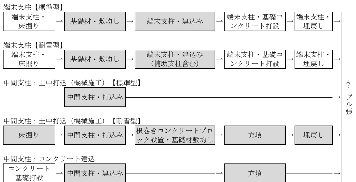
図 2-1 施工フロー
