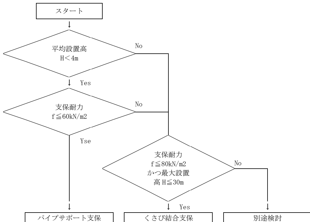
図 2-2 工法の選定
