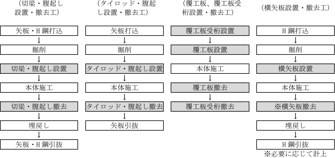
図 2-1 施工フロー
