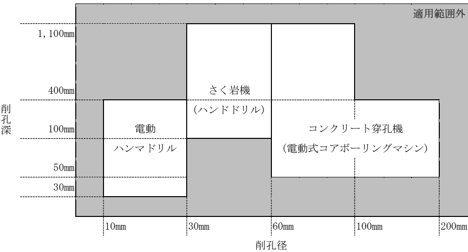
図 1-1 削孔機械の選定
