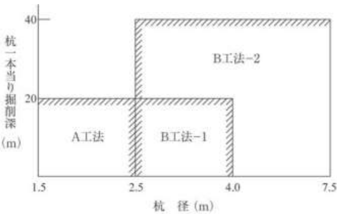
図 1-1 適用杭径及び掘削深（標準）
