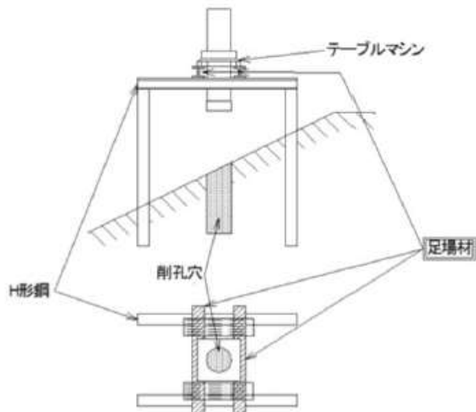
(C工法:作業架台概念図)
