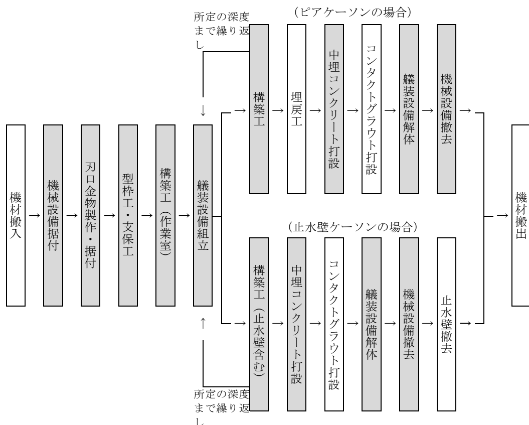
図 2-1 施工フロー
