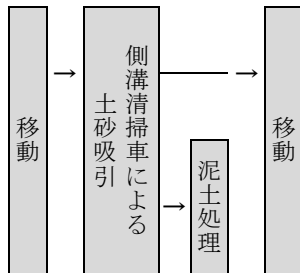
図 2-1 施工フロー
