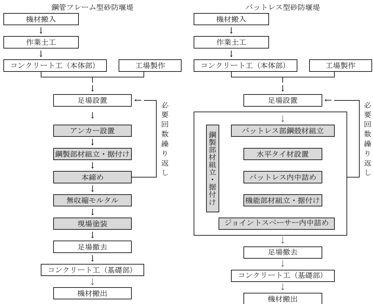
図 2-1 施工フロー
