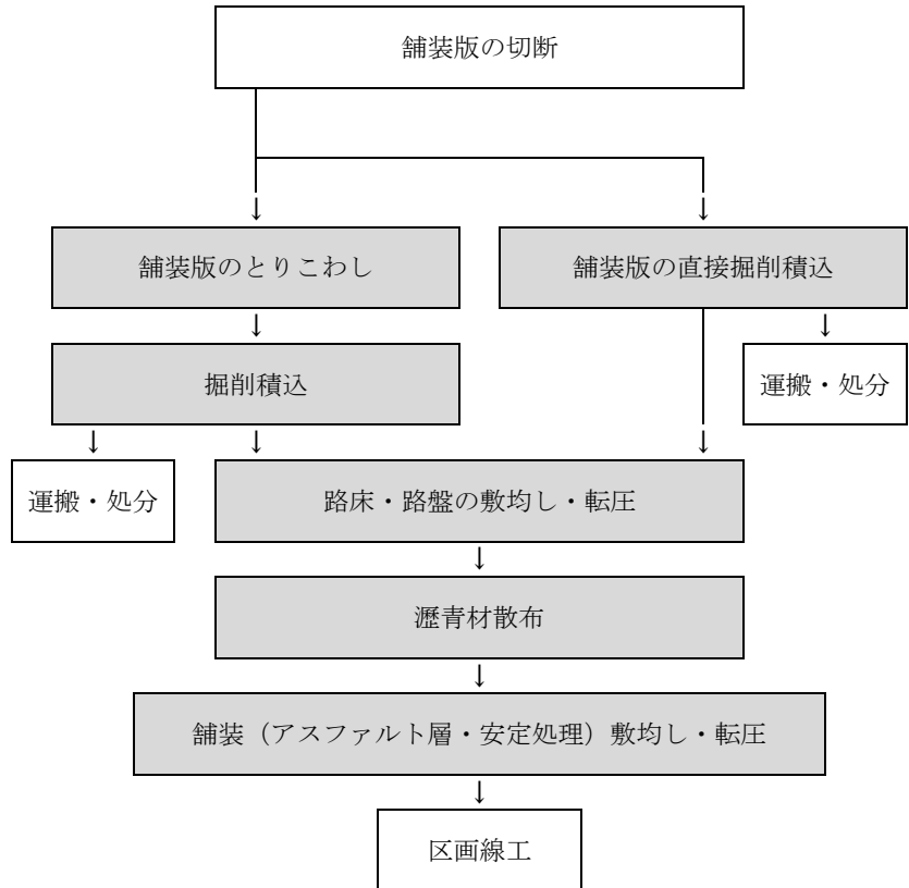
図 2-1 施工フロー
