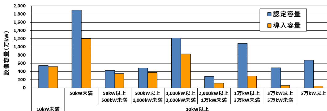
図4 固定価格買取制度における太陽光発電設備の規模別導入・認定状況
