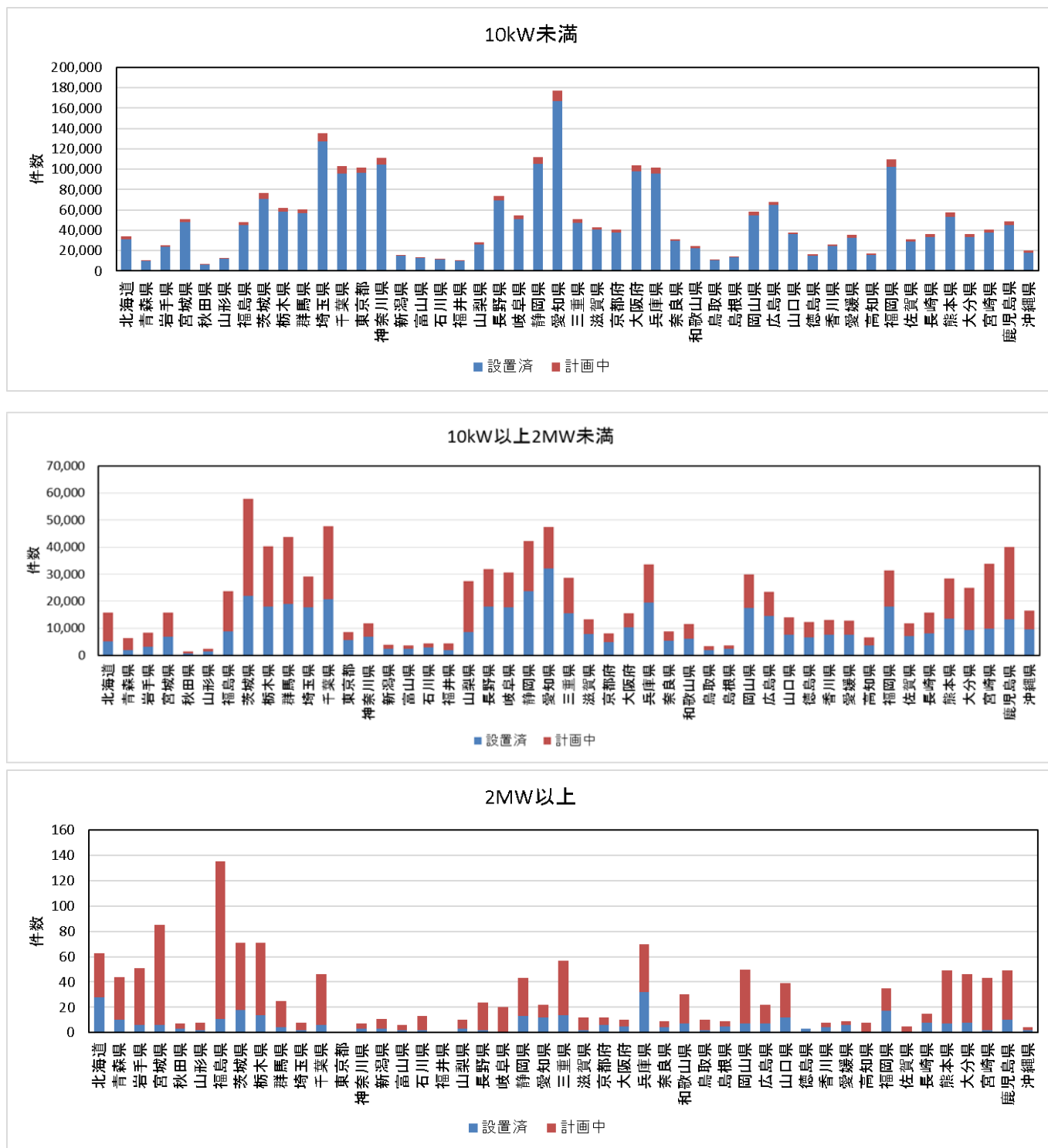
図5 都道府県別・発電出力別の太陽光発電設備の件数
