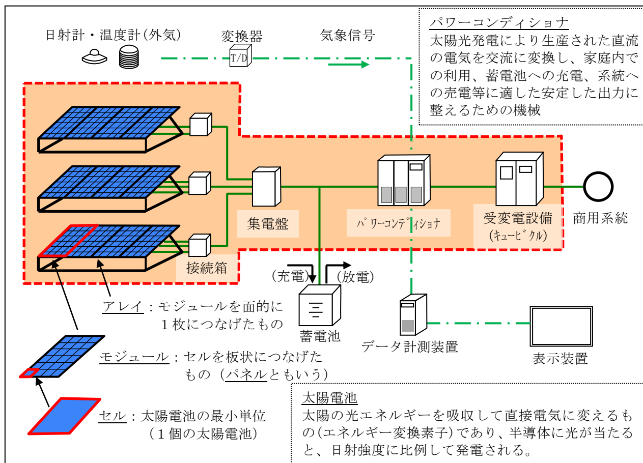
図2 太陽光発電施設の構成の一例
