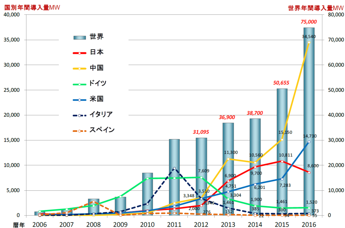
図7 世界の太陽電池設置量の推移（2006-2016）
